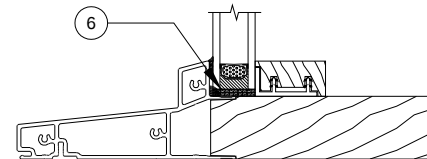
TÊTE ET SEUIL / HEAD AND SILL
