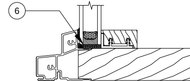
TÊTE ET SEUIL / HEAD AND SILL
