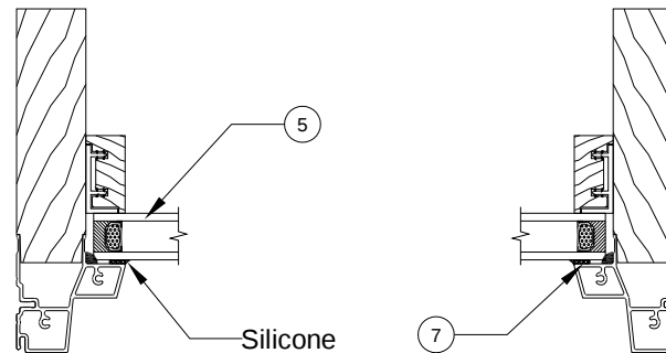
JAMBAGE / JAMB
