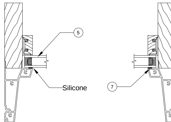
JAMBAGE / JAMB
