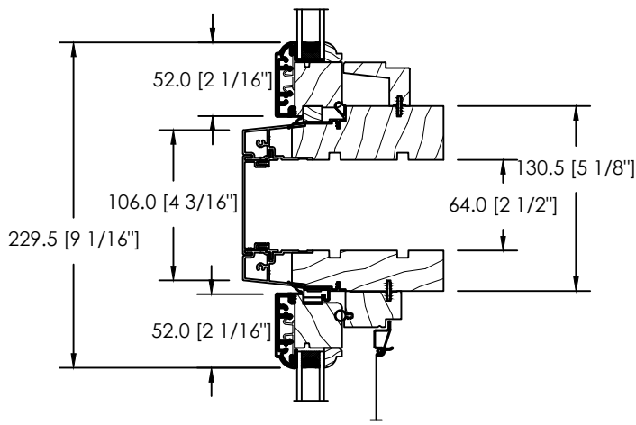
2 1/2" SPACE MULL OR STUD POCKET
