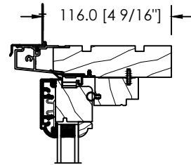
NAILING FIN
