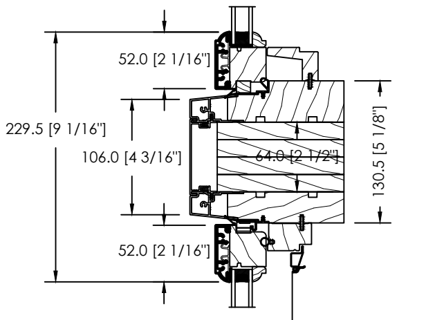
2 1/2" SOLID SPACE MULL OR STUD POCKET
