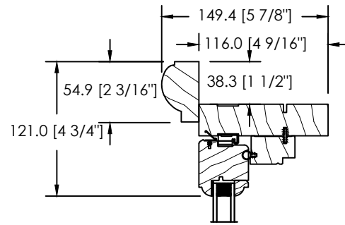
DS-017 BRICKMOULD
