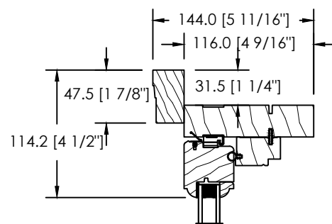
908 BRICKMOULD
