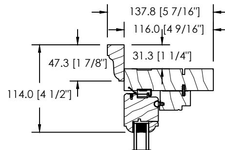
DS-061 BRICKMOULD
