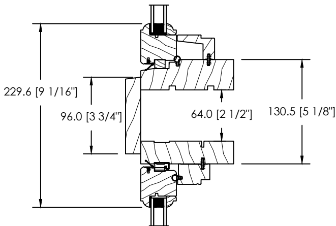
2 1/2" SPACE MULL OR STUD POCKET
