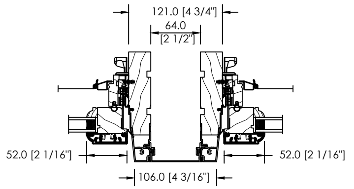
2 1/2" SPACE MULL OR STUD POCKET
