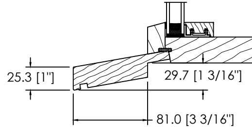
3" SILL EXTENSION (GB-040)
