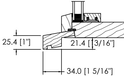
STANDARD SILL EXTENSION (GB-021)
