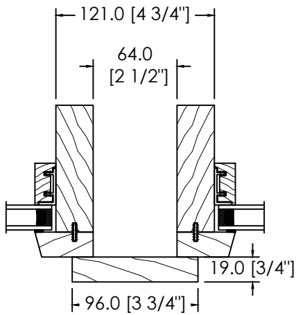
2 1/2" STUD POCKET OR SPACE MULL
