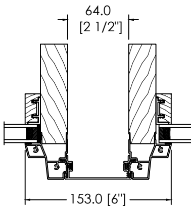
2 1/2" STUD POCKET OR SPACE MULL
