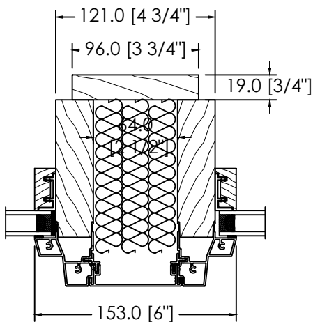
2 1/2" STUD POCKET OR SPACE MULL
