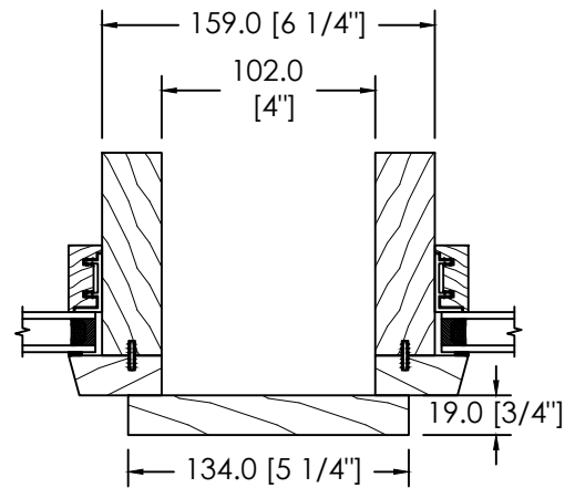
ESPACE MODULAIRE & STRUCTURAL 102MM
