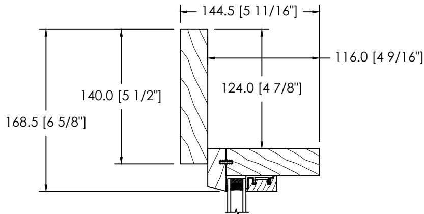
MOULURE À BRIQUE PLATE 140MM D-118
