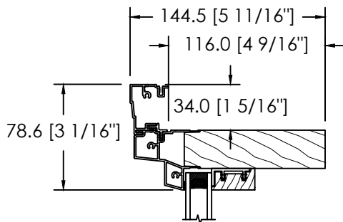
MOULURE À BRIQUE 908
