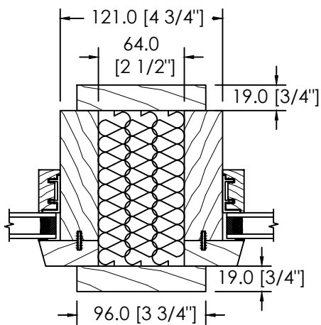
ESPACE MODULAIRE & STRUCTURAL ISOLÉ 64MM
