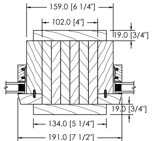
ESPACE MODULAIRE & STRUCTURAL SOLIDE 102MM
