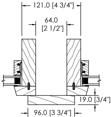
ESPACE MODULAIRE & STRUCTURAL 64MM
