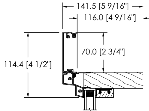
MOULURE À BRIQUE PLATE 70MM D-066
