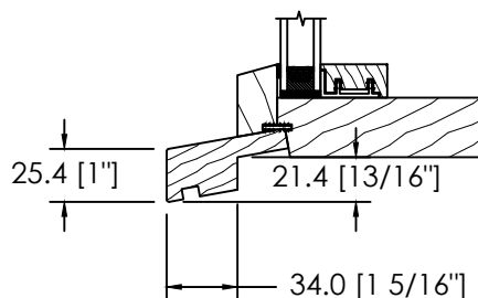
EXTENSION DE SEUIL STANDARD (GB-021)
