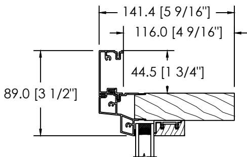
MOULURE À BRIQUE PLATE 44.5MM D-116
