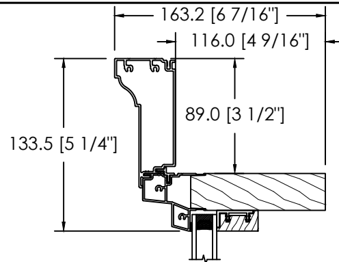
MOULURE À BRIQUE BACK BEND D-090
