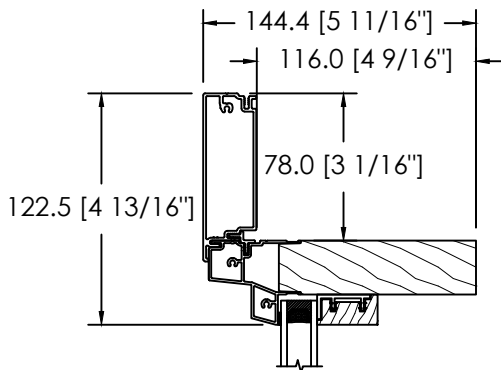
MOULURE À BRIQUE PLATE 89MM D-050
