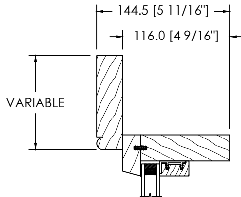
MOULURE À BRIQUE VARIABLE DS-001
