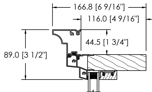
MOULURE À BRIQUE SKYLER D-174
