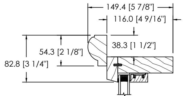
MOULURE À BRIQUE DS-017
