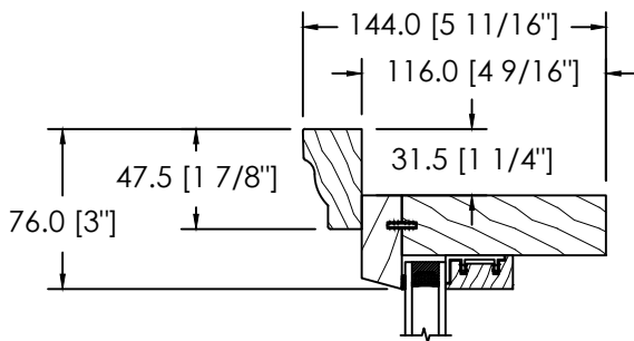
MOULURE À BRIQUE COLONIALE D-017
