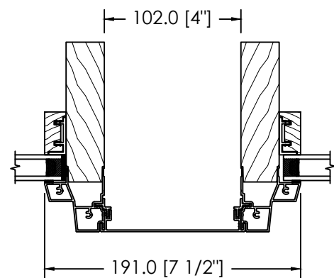
ESPACE MODULAIRE & STRUCTURAL 102MM
