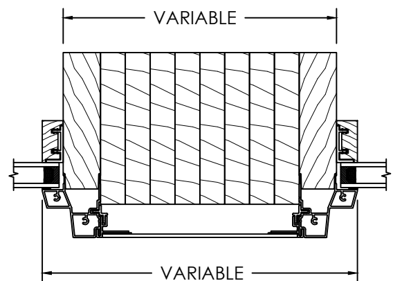
ESPACE MODULAIRE & STRUCTURAL SOLIDE VARIABLE
