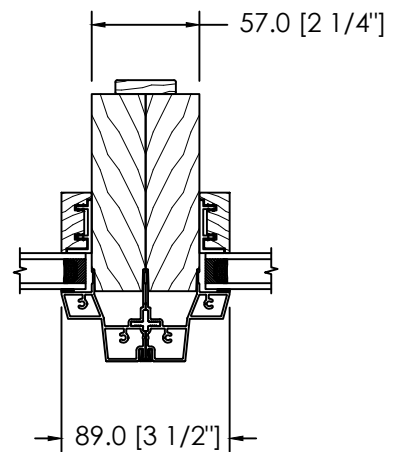
ASSEMBLAGE HORIZONTAL MODULAIRE
