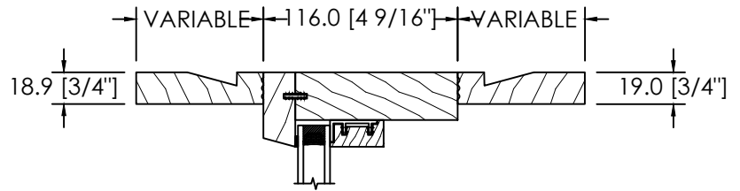
EXTENSION EXT. ET INT. VARIABLE
