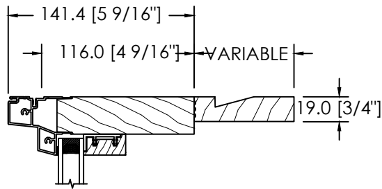
EXTENSION INTÉRIEURE VARIABLE
