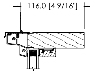
AILE DE CLOUAGE
