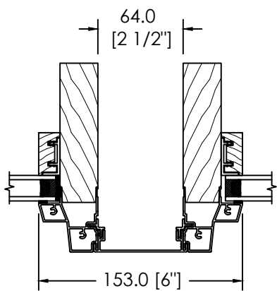
ESPACE MODULAIRE & STRUCTURAL 64MM
