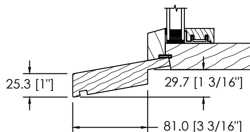
EXTENSION DE SEUIL LONG (GB-040)
