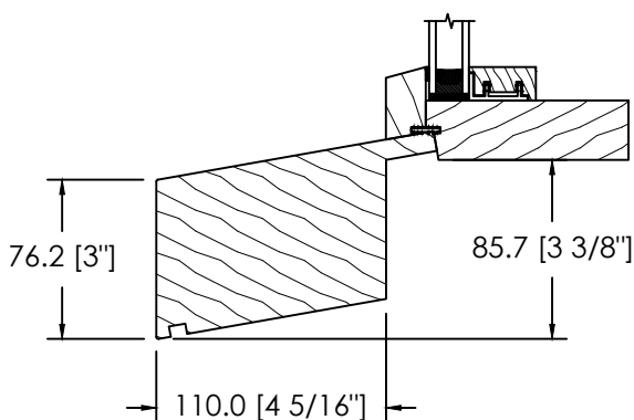
EXTENSION DE SEUIL DS-072
