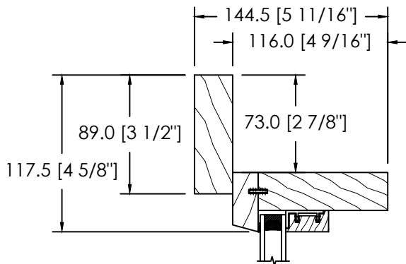
MOULURE À BRIQUE PLATE 89MM D-061
