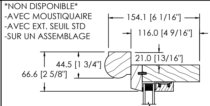
MOULURE À BRIQUE DS-030
