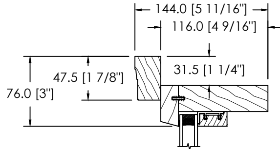
MOULURE À BRIQUE 908 D-064
