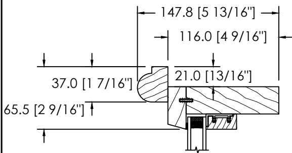
MOULURE À BRIQUE DS-034
