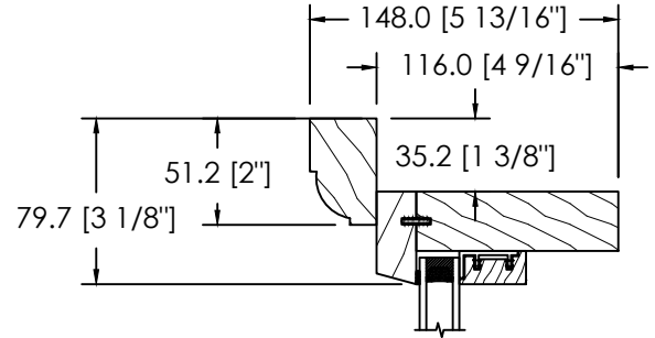
MOULURE À BRIQUE DS-065
