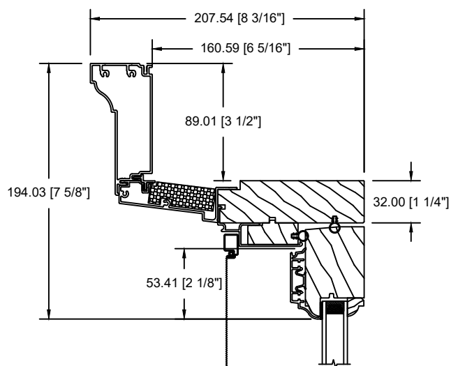
MOULURE À BRIQUE BACKBEND 3 15/16" (D-090)
