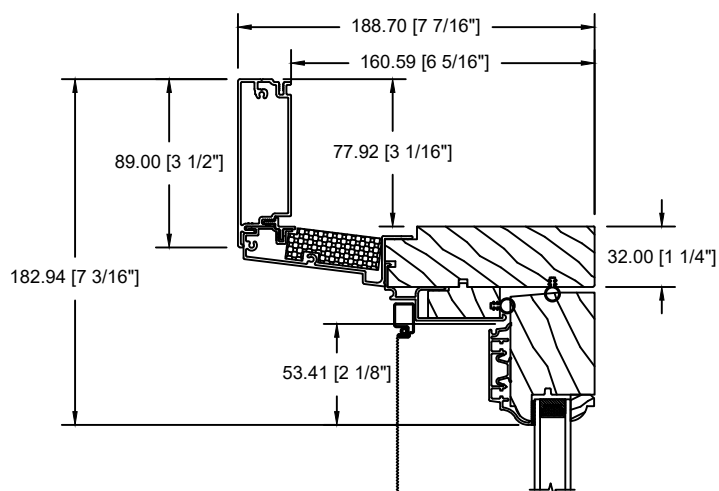
MOULURE À BRIQUE PLATE 3 1/2" (D-050)
