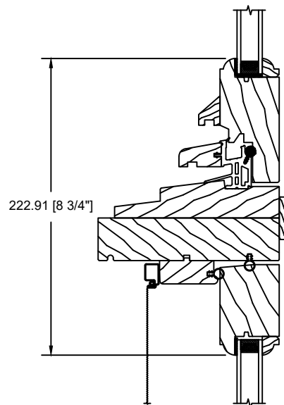
IMPOSTE AVEC VOLET
