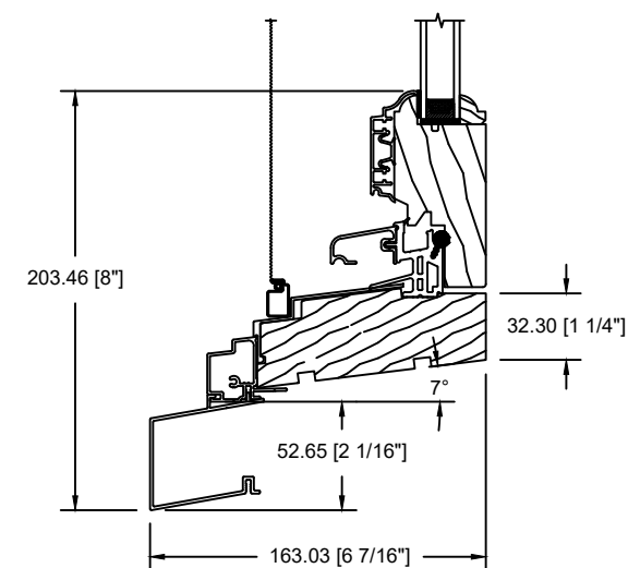
EXTENSION SEUIL HISTORIQUE
