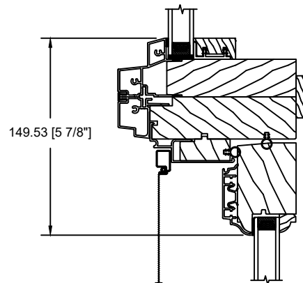
IMPOSTE THERMO FIXE
