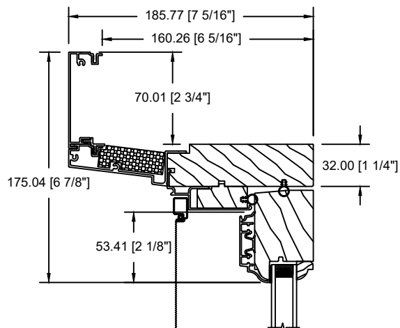
MOULURE À BRIQUE PLATE 2 3/4"
