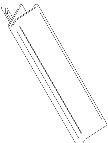
CF-006 COUPE-FROID POLYFLEX / POLYFLEX WEATHER STRIP SUR LE VOLET DE BOIS / ON WOOD SASH
