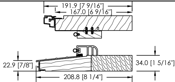
CADRE 116mm - SEUIL ANODISÉ
