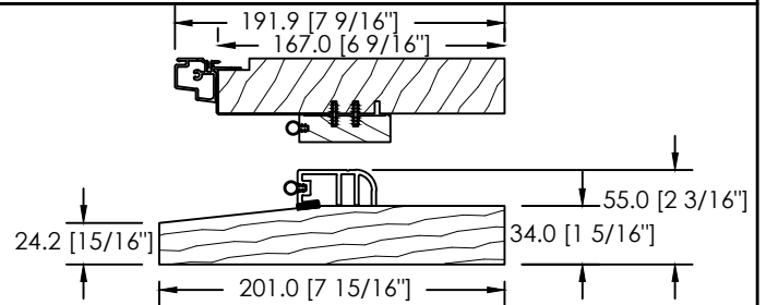
CADRE 116mm - SEUIL EN ACAJOU
