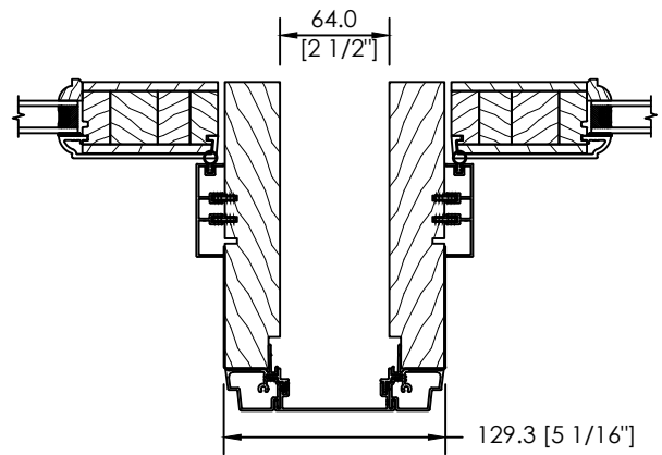
ESPACE MODULAIRE OU STRUCTURAL STANDARD 64mm
