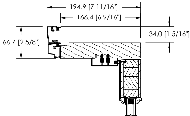
MOULURE À BRIQUE 908
