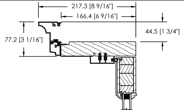
MOULURE À BRIQUE SKYLER D-174
