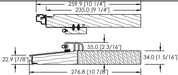
CADRE 235mm - SEUIL ANODISÉ
