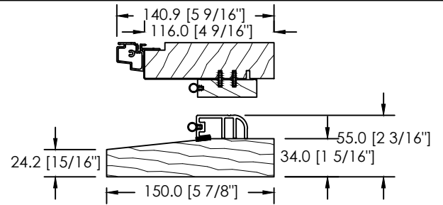
CADRE 116mm - SEUIL EN ACAJOU
