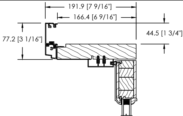
MOULURE À BRIQUE PLATE 44.5MM D-116
