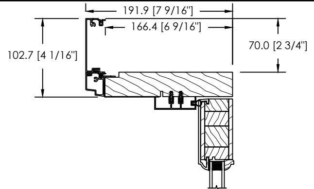
MOULURE À BRIQUE PLATE 70MM D-066
