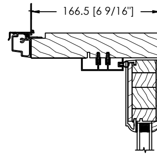
AILE DE CLOUAGE
