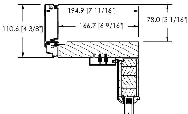
MOULURE À BRIQUE PLATE 89MM D-050
