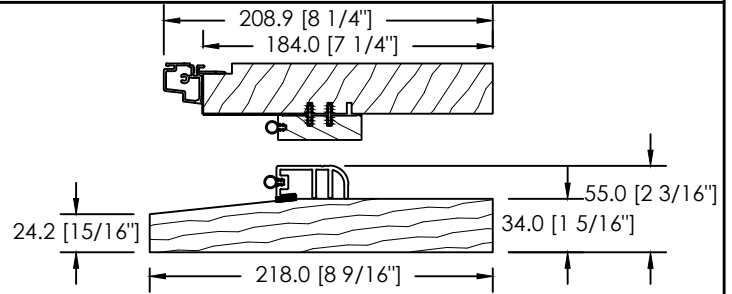
CADRE 167mm - SEUIL EN ACAJOU
