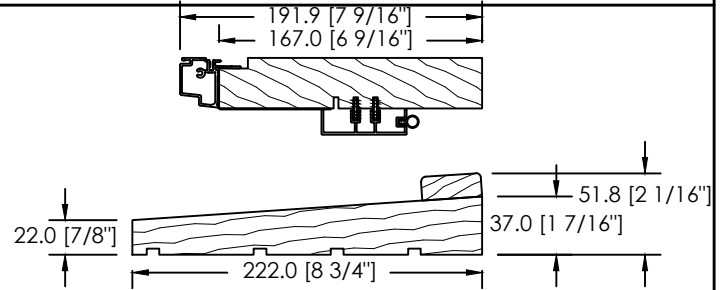
CADRE 167mm - SEUIL EN ACAJOU BRIS THERMIQUE EN ACAJOU
