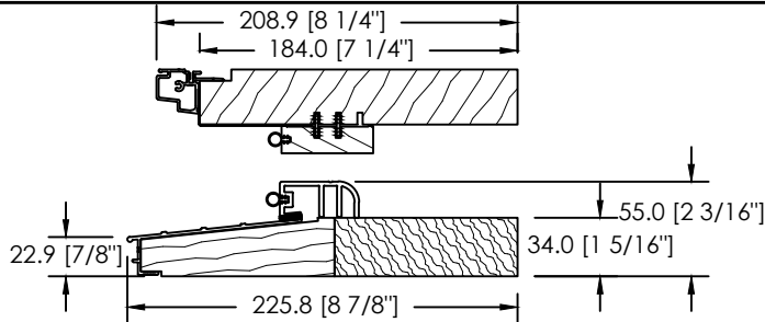
CADRE 167mm - SEUIL ANODISÉ
