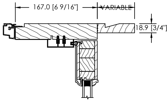
EXTENSION INTÉRIEURE VARIABLE
