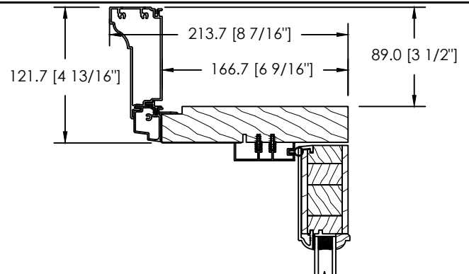
MOULURE À BRIQUE BACK BEND D-090
