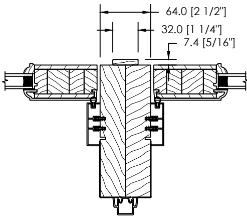
ASSEMBLAGE VERTICAL MODULAIRE
