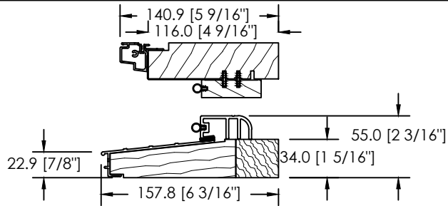
CADRE 116mm - SEUIL ANODISÉ
