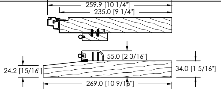
CADRE 235mm - SEUIL EN ACAJOU
