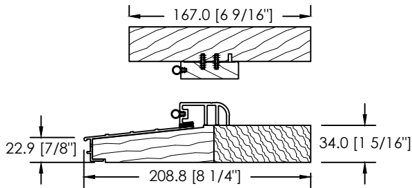
CADRE 167mm - SEUIL ANODISÉ
