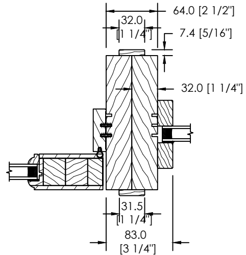
ASSEMBLAGE VERTICAL MODULAIRE AVEC THERMOS FIXE (SL-1)
