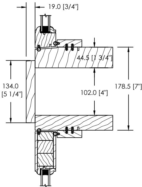
ESPACE MODULAIRE OU STRUCTURAL STANDARD 102mm
