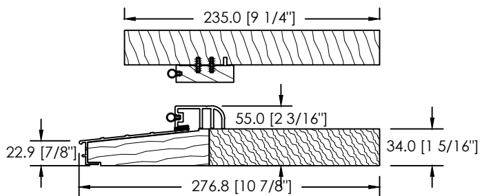
CADRE 235mm - SEUIL ANODISÉ
