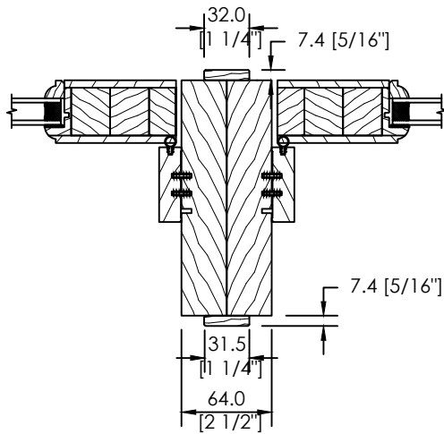
ASSEMBLAGE VERTICAL MODULAIRE
