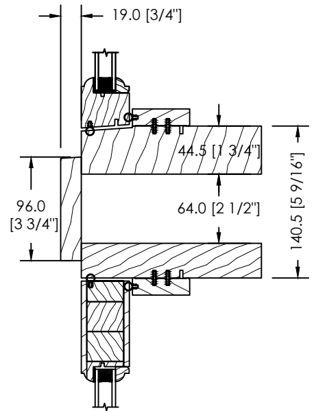
ESPACE MODULAIRE OU STRUCTURAL STANDARD 64mm
