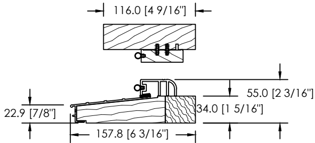
CADRE 116mm - SEUIL ANODISÉ
