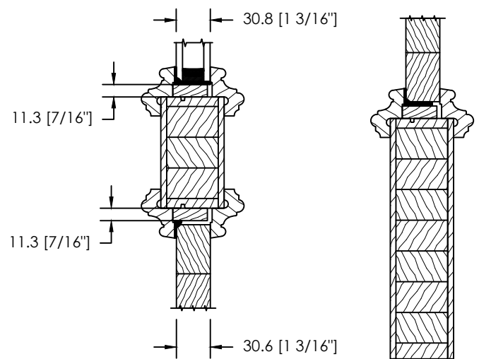
MOULURE DÉCORATIVE CONTEMPORAINE D-181 AVEC PANNEAU PLAT
