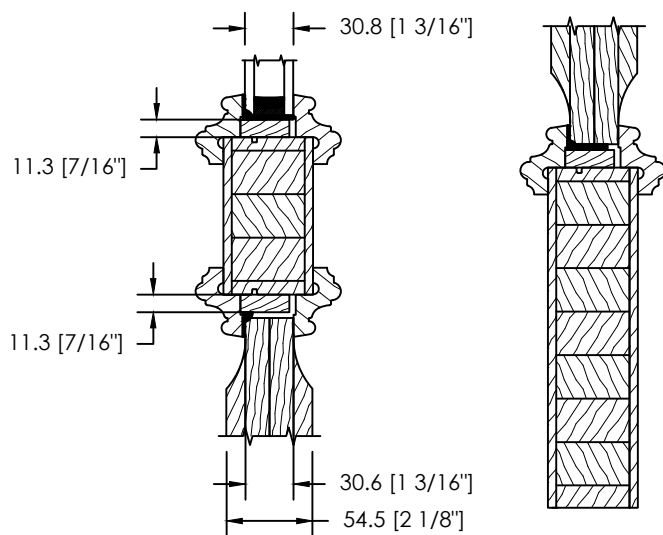
MOULURE DÉCORATIVE CONTEMPORAINE D-181 AVEC PANNEAU RAVALÉ
