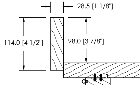
MOULURE À BRIQUE 908
