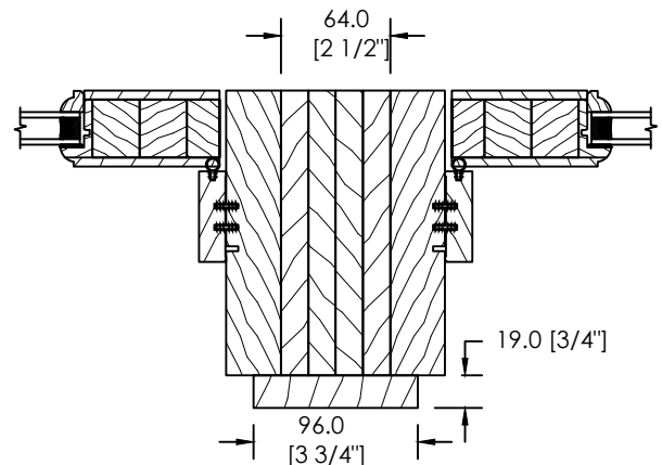
ESPACE MODULAIRE OU STRUCTURAL SOLIDE - STANDARD 64mm
