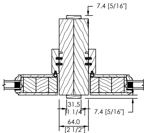
ASSEMBLAGE VERTICAL MODULAIRE
