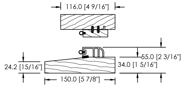
CADRE 116mm - SEUIL EN ACAJOU
