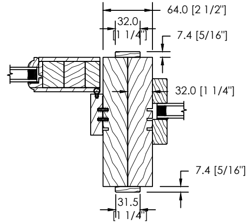
ASSEMBLAGE VERTICAL MODULAIRE AVEC THERMOS FIXE (SL-1)
