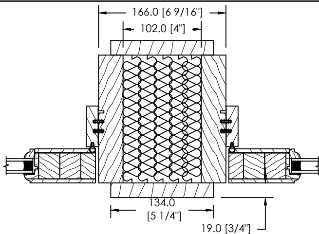
ESPACE MODULAIRE OU STRUCTURAL ISOLÉ - STANDARD 102mm
