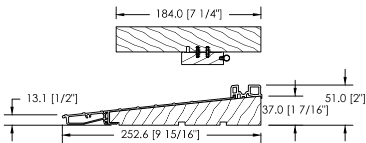
CADRE 184mm - SEUIL ANODISÉ + EXT. 2" BRIS THERMIQUE EN PVC
