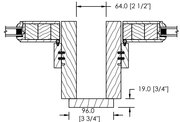
ESPACE MODULAIRE OU STRUCTURAL STANDARD 64mm
