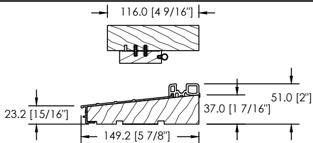
CADRE 116mm - SEUIL ANODISÉ BRIS THERMIQUE EN PVC
