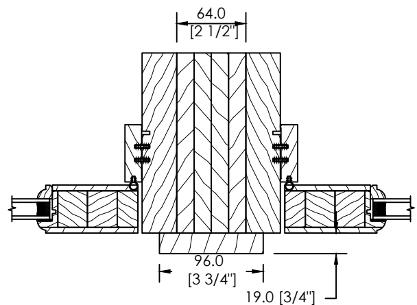
ESPACE MODULAIRE OU STRUCTURAL SOLIDE - STANDARD 64mm
