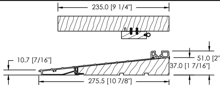
CADRE 235mm - SEUIL ANODISÉ + EXT. 3" BRIS THERMIQUE EN PVC
