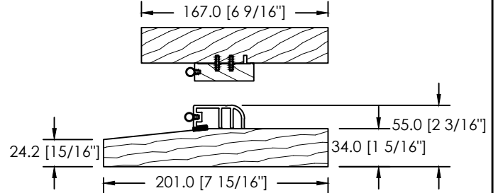
CADRE 167mm - SEUIL EN ACAJOU
