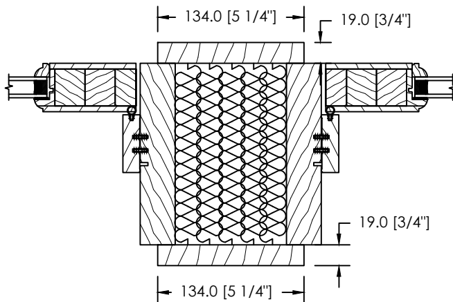
ESPACE MODULAIRE OU STRUCTURAL ISOLÉ - STANDARD 102mm
