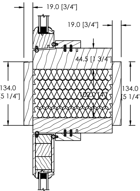
ESPACE MODULAIRE OU STRUCTURAL ISOLÉ - STANDARD 102mm
