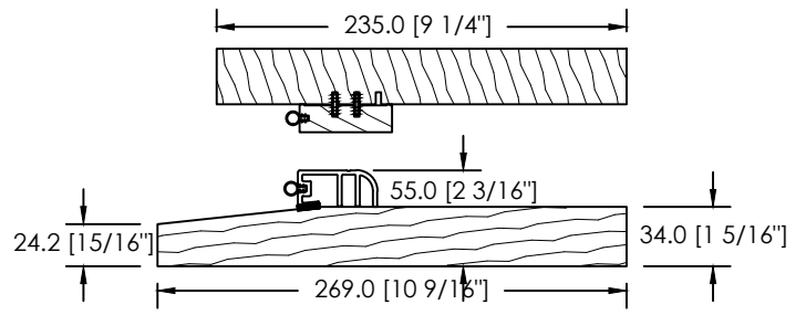
CADRE 235mm - SEUIL EN ACAJOU
