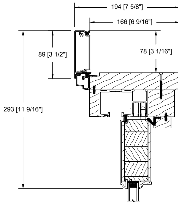
MOULURE À BRIQUE PLATE 3 \frac{1}{2} \"/>
