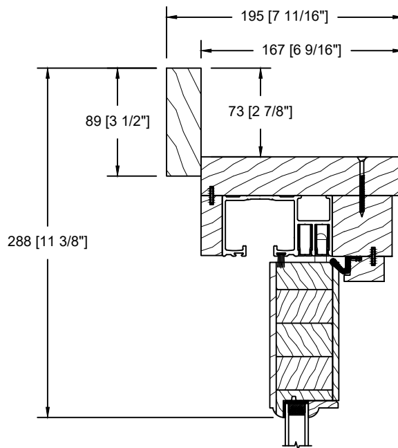
MOULURE À BRIQUE PLATE 3 ½"
