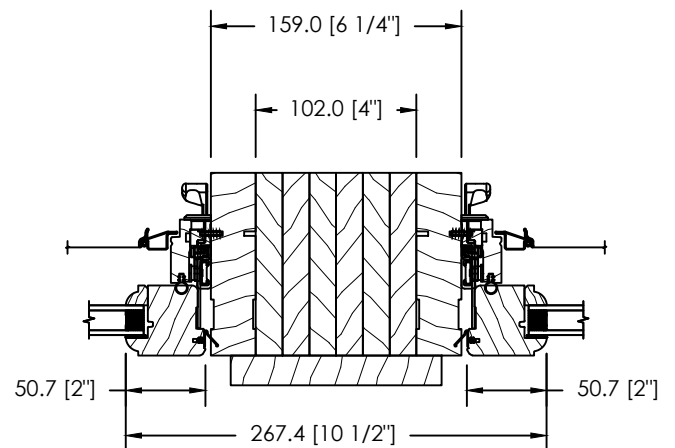
ESPACE MODULAIRE & STRUCTURAL SOLIDE 102MM
