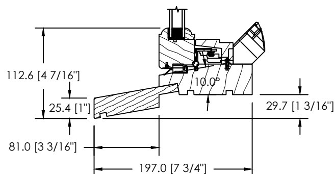
EXTENSION DE SEUIL LONG GB-040
