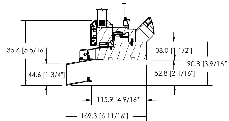
EXTENSION DE SEUIL HISTORIQUE D-083
