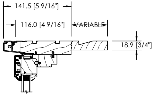
EXTENSION INTÉRIEURE VARIABLE
