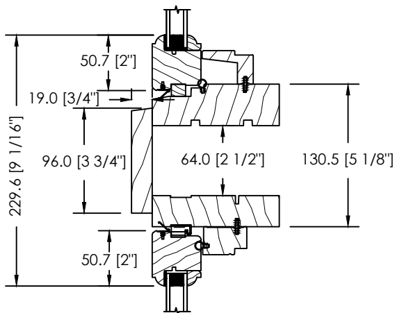
ESPACE MODULAIRE & STRUCTURAL 64MM
