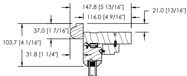
MOULURE À BRIQUE DS-034
