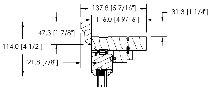
MOULURE À BRIQUE DS-061
