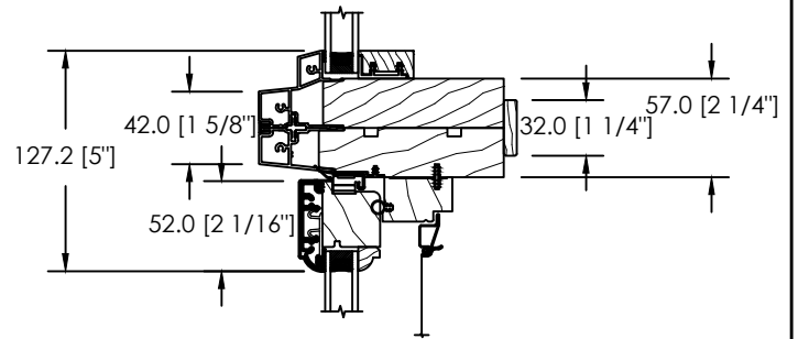
IMPOSTE THERMOS FIXE
