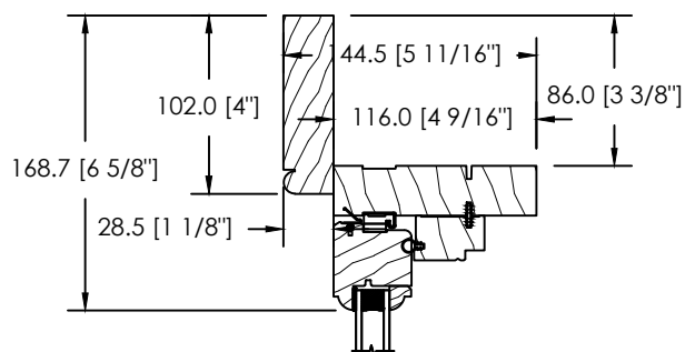
MOULURE À BRIQUE DS-001
