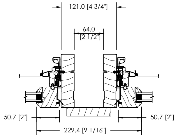
OUVRANT ET THERMOS FIXE
