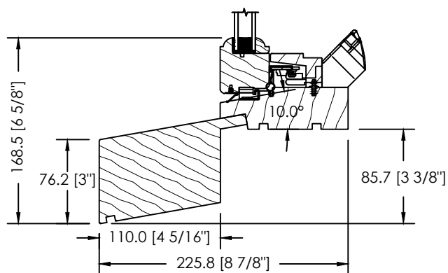
EXTENSION DE SEUIL DS-072
