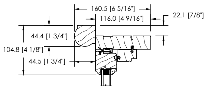
MOULURE À BRIQUE DS-030
