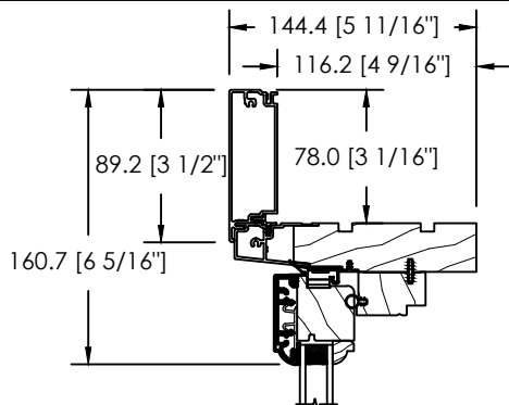
MOULURE À BRIQUE PLATE 89MM D-050
