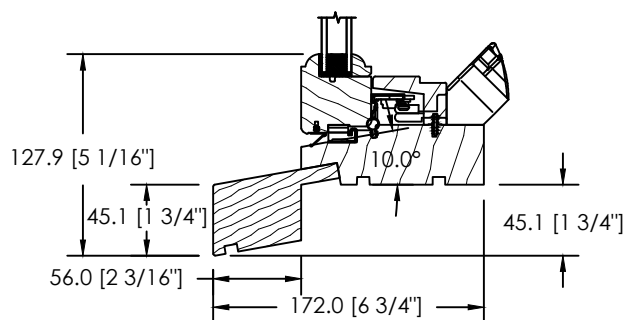
EXTENSION DE SEUIL HISTORIQUE GB-036
