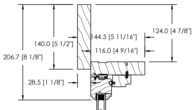
MOULURE À BRIQUE PLATE 140MM
