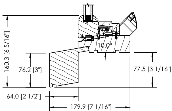
EXTENSION DE SEUIL DS-073
