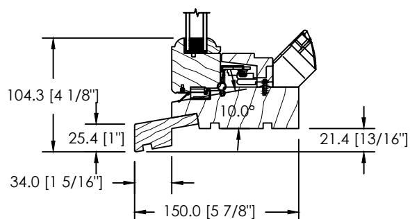
EXTENSION DE SEUIL STANDARD GB-021
