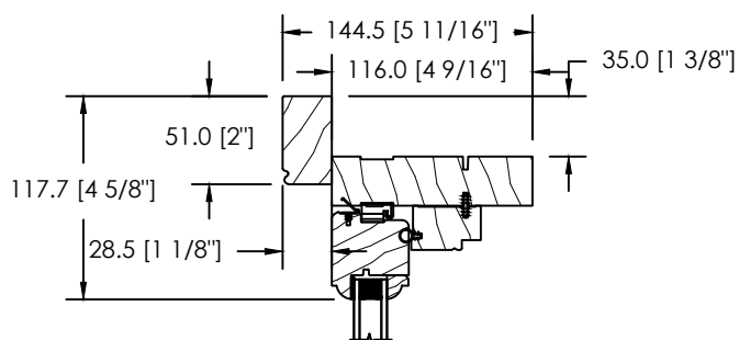
MOULURE À BRIQUE DS-031
