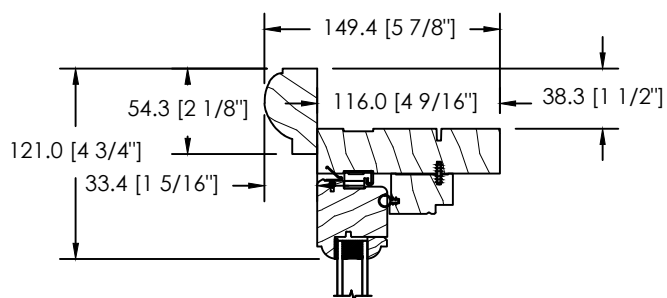
MOULURE À BRIQUE DS-017
