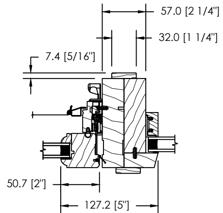
OUVRANT ET THERMOS FIXE
