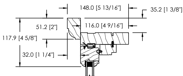
MOULURE À BRIQUE DS-065
