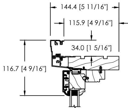
MOULURE À BRIQUE 908
