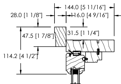
MOULURE À BRIQUE 908
