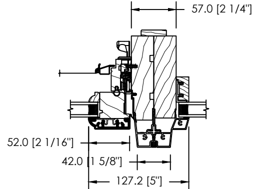
OUVRANT ET THERMOS FIXE
