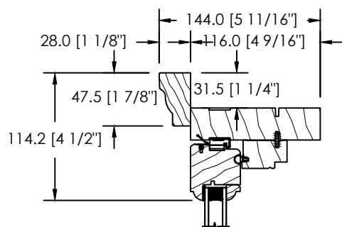
MOULURE À BRIQUE COLONIALE
