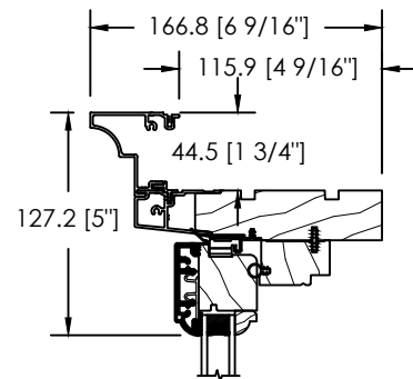
MOULURE À BRIQUE SKYLER D-174
