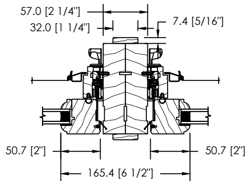
2 OUVRANTS - ASSEMBLAGE MODULAIRE
