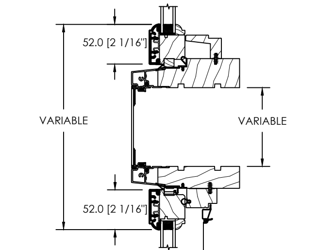
ESPACE MODULAIRE & STRUCTURAL NON-STANDARD 8" MAXIMUM
