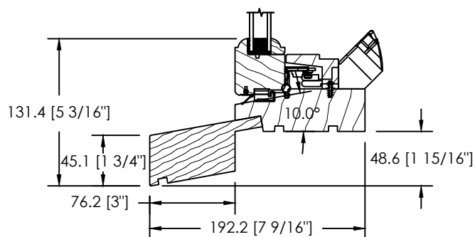
EXTENSION DE SEUIL HISTORIQUE LONG GB-058
