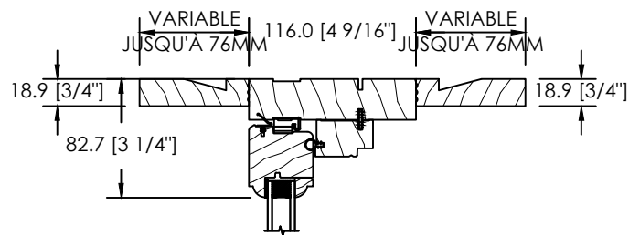
EXTENSION EXT. ET INT. VARIABLE
