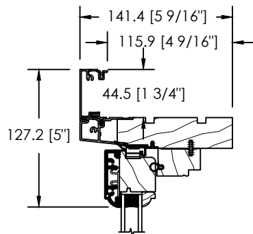
MOULURE À BRIQUE PLATE 44.5MM D-116
