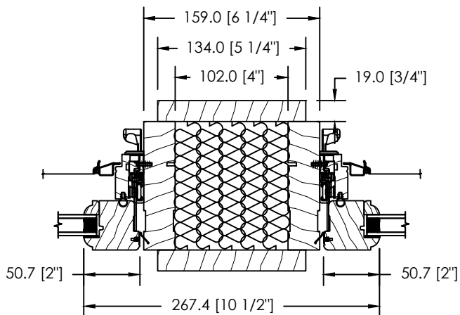
ESPACE MODULAIRE & STRUCTURAL ISOLÉ 102MM
