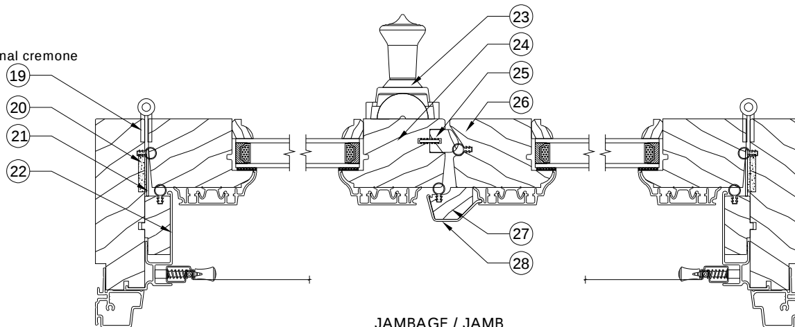
JAMBAGE / JAMB
