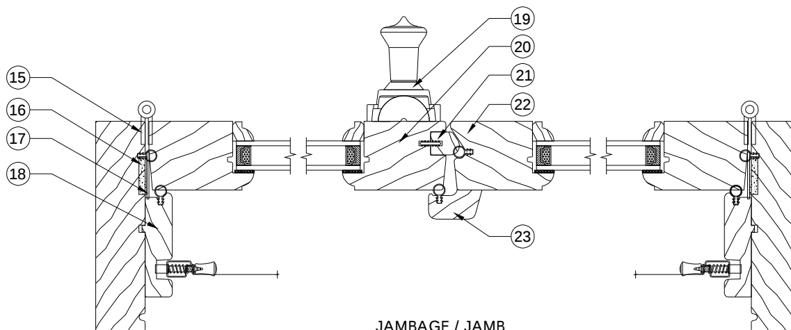
JAMBAGE / JAMB
