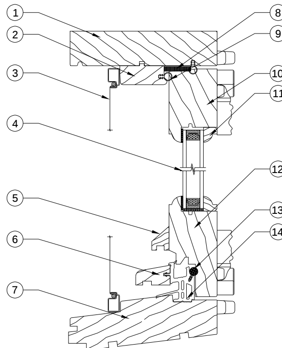
TÊTE ET SEUIL / HEAD AND SILL
