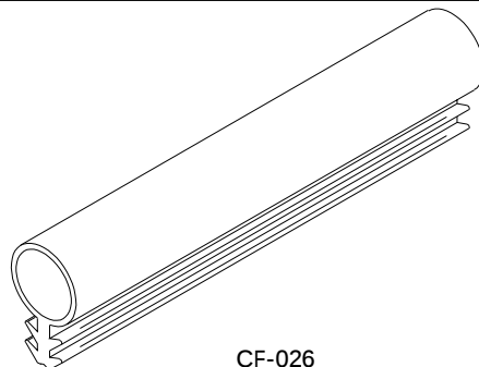
CF-026 COUPE-FROID SILICONE / SILOCONE WEATHER STRIP SUR LE CADRE, L'ASTRAGALE ET LA RENCONTRE DE VOLET / ON FRAME, ASTRAGALE AND MEETING RAIL
