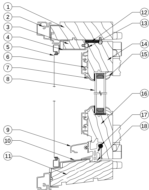
TÊTE ET SEUIL / HEAD AND SILL
