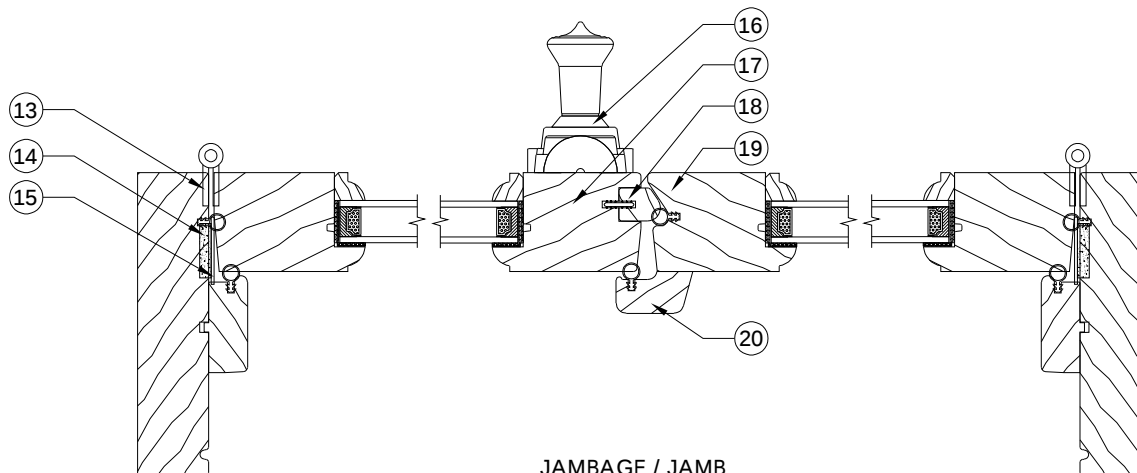
JAMBAGE / JAMB
