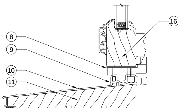
TÊTE ET SEUIL / HEAD AND SILL
