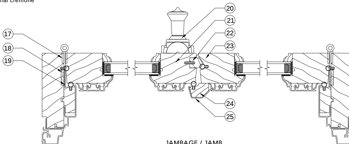
JAMBAGE / JAMB
