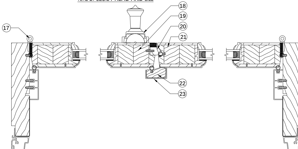
TÊTE ET SEUIL / HEAD AND SILL
