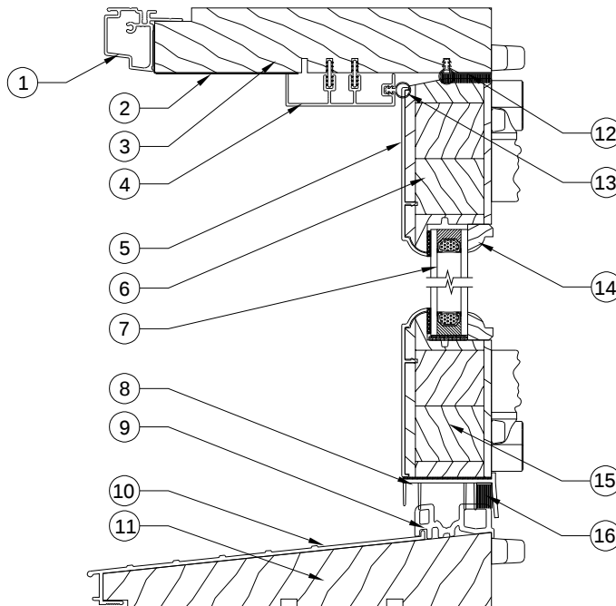
TÊTE ET SEUIL / HEAD AND SILL
