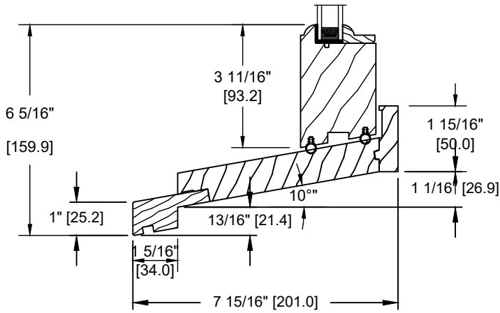
STANDARD SILL EXTENSION (GB-021)
