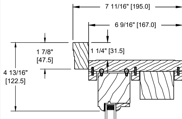
908 BRICKMOULD (D-064)
