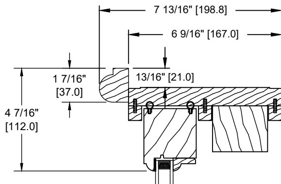
SPECIAL BRICKMOULD (DS-034)
