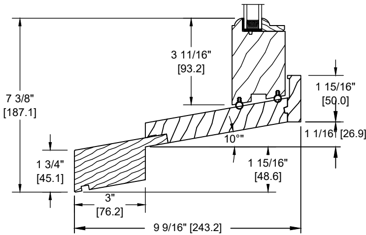
HISTORIC SILL EXTENSION (GB-058)
