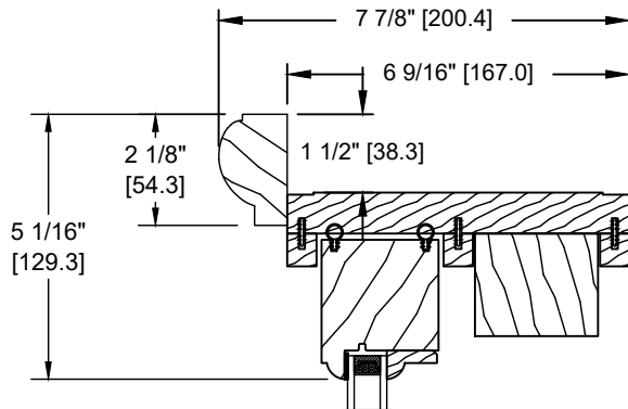
SPECIAL BRICKMOULD (DS-017)
