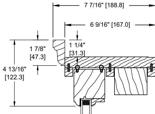
SPECIAL BRICKMOULD (DS-061)
