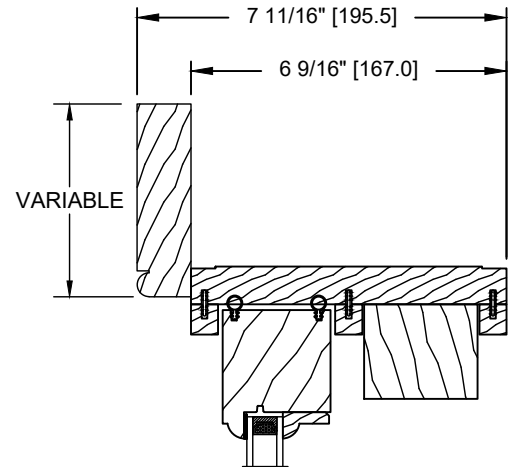
VARIABLE BRICKMOULD (DS-001)
