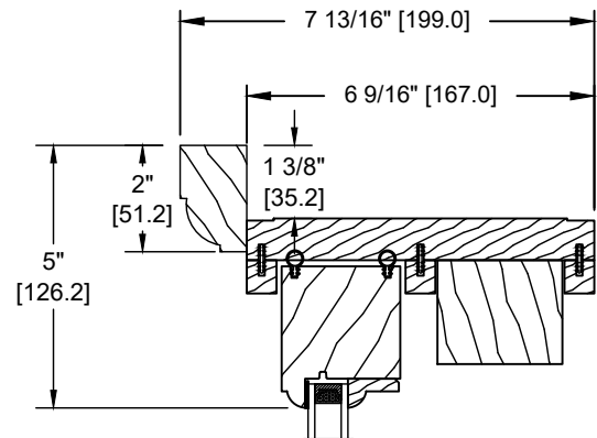
SPECIAL BRICKMOULD (DS-065)
