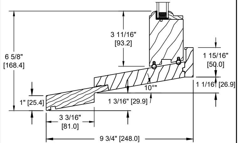
3" SILL EXTENSION (GB-040)
