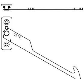
Q-264 LIMITEUR D'OUVERTURE À DÉGAGEMENT RAPIDE / FAST RELEASE SASH LIMITER
