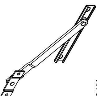
Q-122 LIMITEUR D'OUVERTURE STANDARD / STANDARD LIMIT DEVICE
