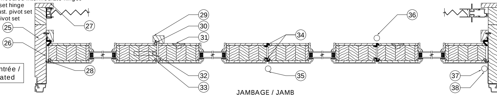
JAMBAGE / JAMB
