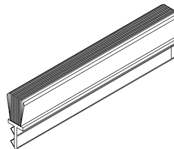
CF-029 COUPE-FROID / WEATHER STRIP SOUS LE VOLET / UNDER SASH
