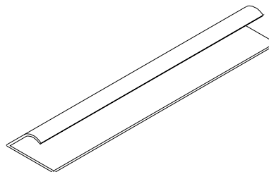
CF-034 COUPE-FROID / WEATHER STRIP SUR LE VOLET (REC. ALUM.) / ON SASH (ALUM. CLAD)
