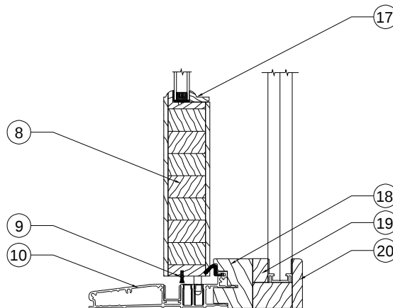
TÊTE ET SEUIL / HEAD AND SILL
