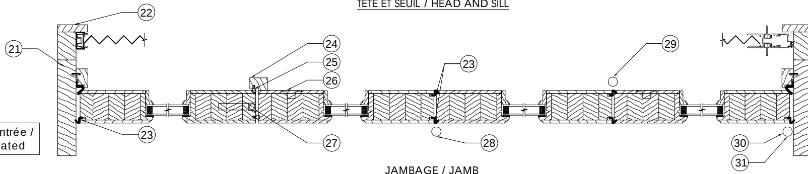
JAMBAGE / JAMB
