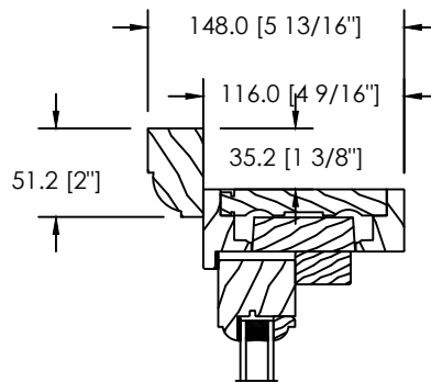
SPECIAL BRICKMOULD (DS-065)
