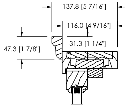
SPECIAL BRICKMOULD (DS-061)
