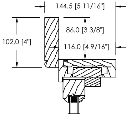
VARIABLE BRICKMOULD (DS-001)
