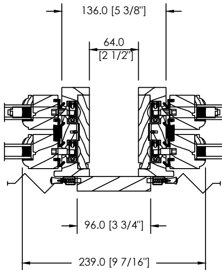
2 1/2" SPACE MULL OR STUD POCKET
