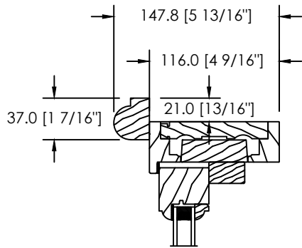
SPECIAL BRICKMOULD (DS-034)
