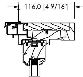
NAILING FIN
