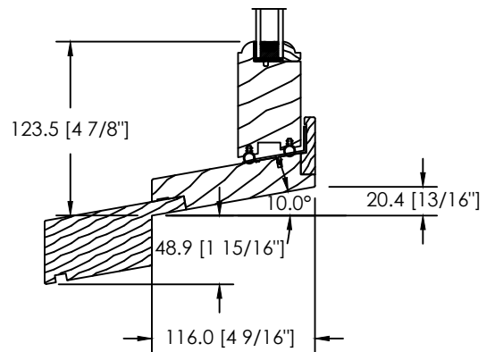
HISTORIC SILL EXTENSION (GB-058)
