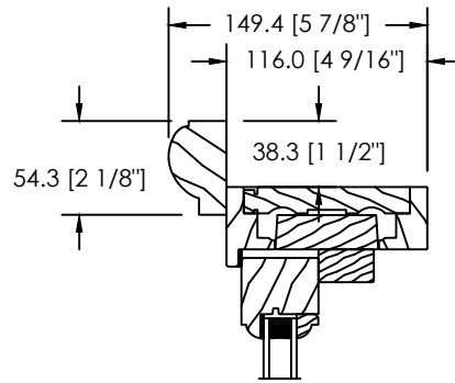
SPECIAL BRICKMOULD (DS-017)
