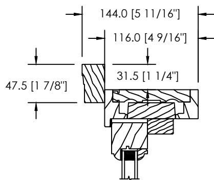
MOULURE À BRIQUE 908 (D-064)
