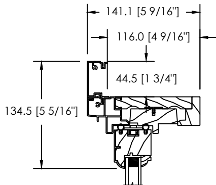
MOULURE À BRIQUE PLATE 44.5MM
