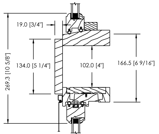
ESPACE MODULAIRE OU STUD POCKET 102MM
