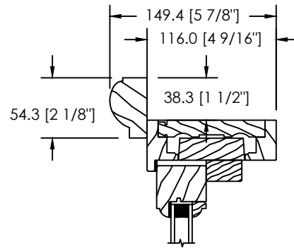
MOULURE À BRIQUE SPÉCIALE (DS-017)
