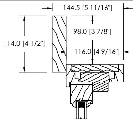
MOULURE À BRIQUE PLATE 114MM (D-117)
