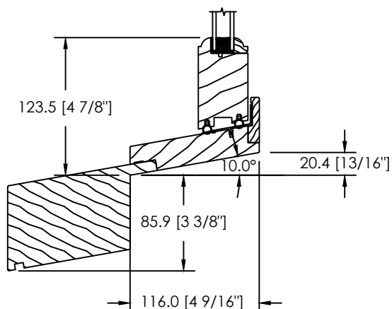
EXTENSION DE SEUIL SPÉCIALE (DS-072)
