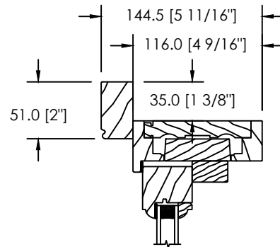
MOULURE À BRIQUE SPÉCIALE (DS-031)
