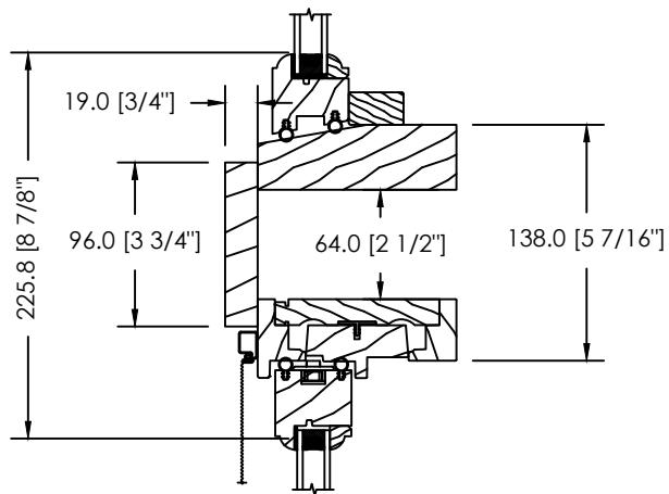
ESPACE MODULAIRE OU STUD POCKET 64MM
