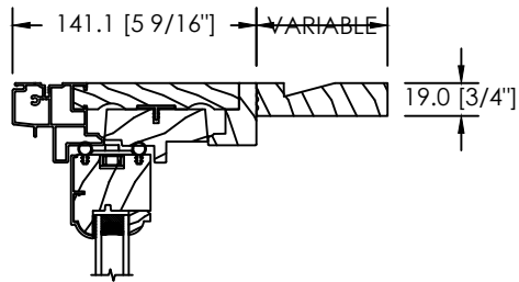
EXTENSION INTÉRIEUR VARIABLE
