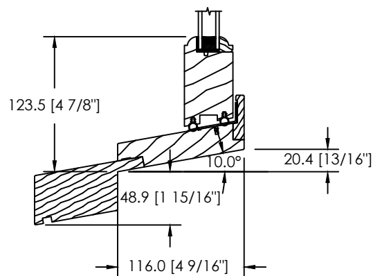
EXTENSION DE SEUIL HISTORIQUE (GB-058)
