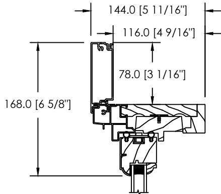
MOULURE À BRIQUE PLATE 89MM
