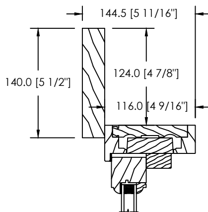
MOULURE À BRIQUE PLATE 140MM (D-118)
