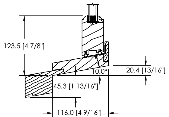
EXTENSION DE SEUIL HISTORIQUE (GB-036)
