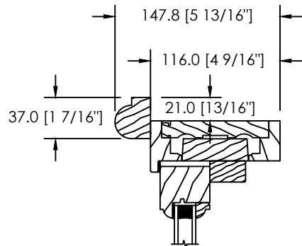
MOULURE À BRIQUE SPÉCIALE (DS-034)
