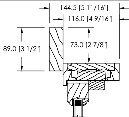
MOULURE À BRIQUE PLATE 89MM (D-061)
