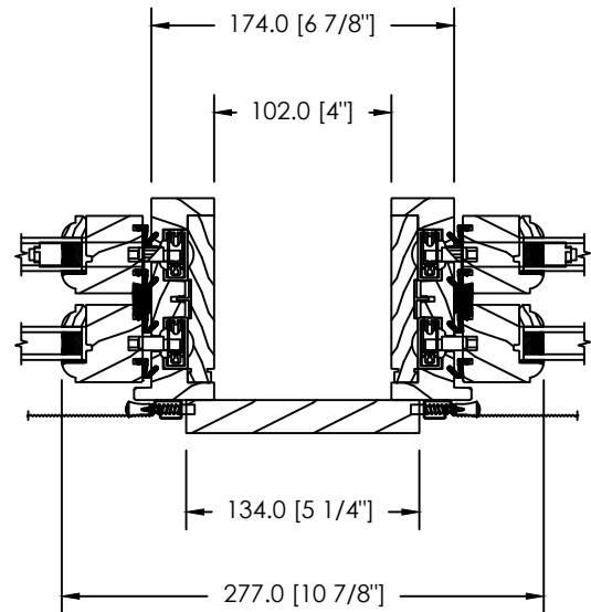
ESPACE MODULAIRE OU STUD POCKET 102MM
