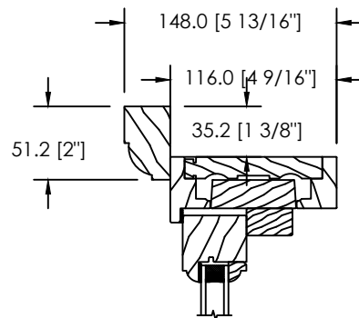
MOULURE À BRIQUE SPÉCIALE (DS-065)
