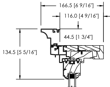
MOULURE À BRIQUE SKYLER
