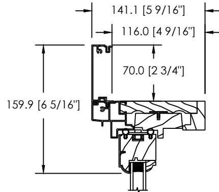
MOULURE À BRIQUE PLATE 70MM
