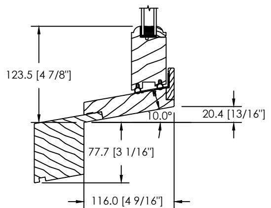
EXTENSION DE SEUIL SPÉCIALE (DS-073)
