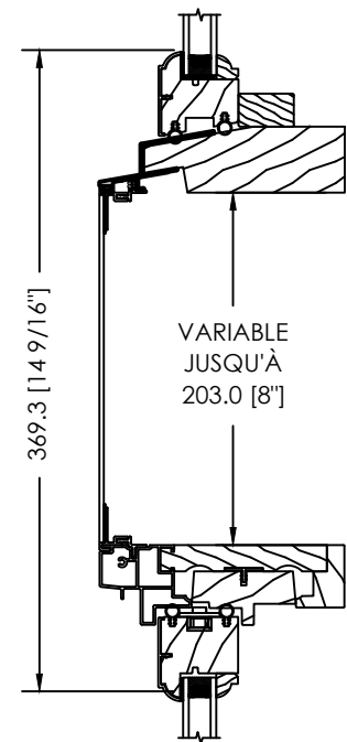
ESPACE MODULAIRE OU STUD POCKET NON STANDARD JUSQU'À 203MM MAXIMUM
