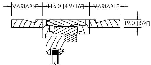
EXTENSION EXT. ET INT. VARIABLE
