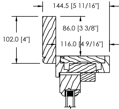
MOULURE À BRIQUE VARIABLE (DS-001)
