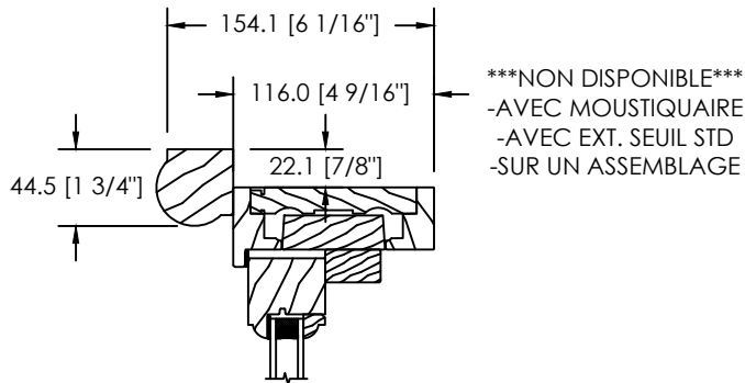
MOULURE À BRIQUE SPÉCIALE (DS-030)
