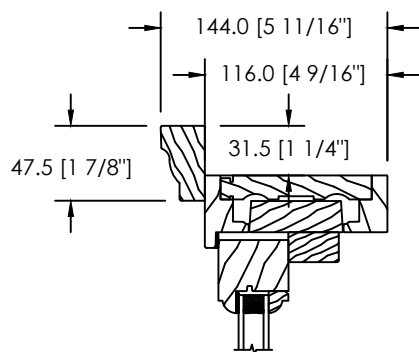
MOULURE À BRIQUE COLONIALE (D-017)
