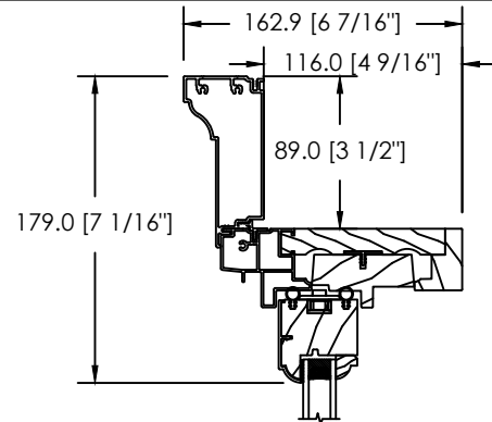
MOULURE À BRIQUE BACK BEND
