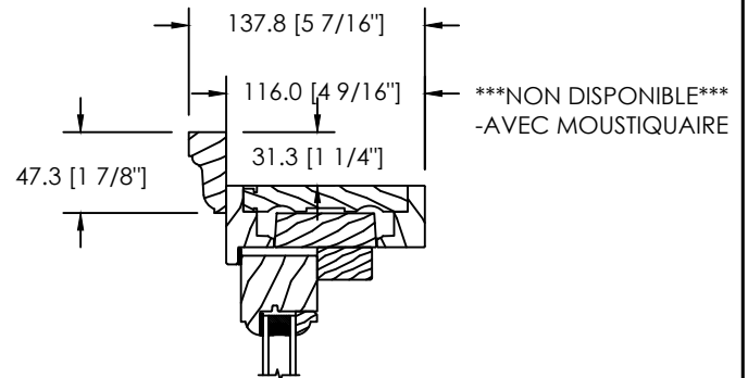
MOULURE À BRIQUE SPÉCIALE (DS-061)
