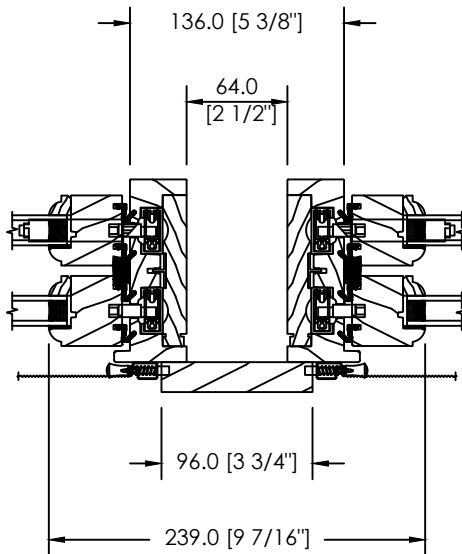
ESPACE MODULAIRE OU STUD POCKET 64MM
