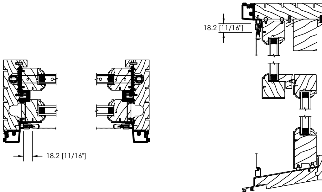
MOUSTIQUAIRE STANDARD
