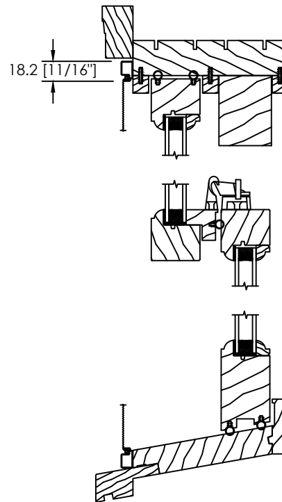
MOUSTIQUAIRE STANDARD
