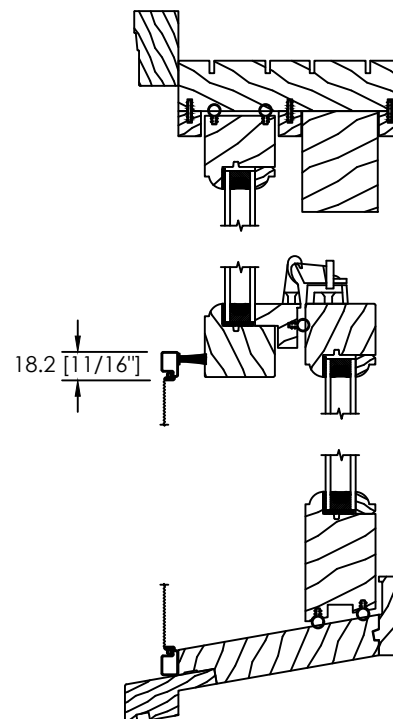
OPTION DEMI-MOUSTIQUAIRE
