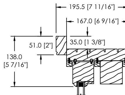
MOULURE À BRIQUE SPÉCIALE (DS-031)
