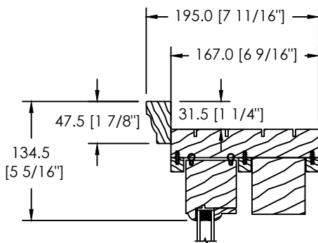
MOULURE À BRIQUE COLONIALE (D-017)
