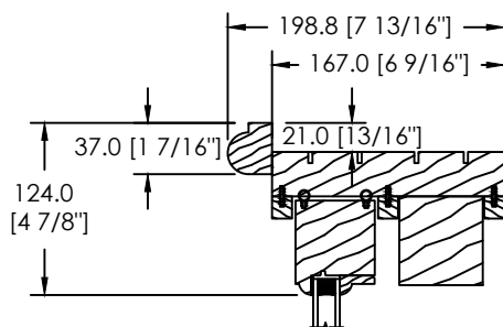
MOULURE À BRIQUE SPÉCIALE (DS-034)
