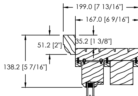
MOULURE À BRIQUE SPÉCIALE (DS-065)
