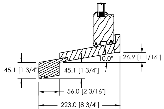
EXTENSION DE SEUIL HISTORIQUE (GB-036)
