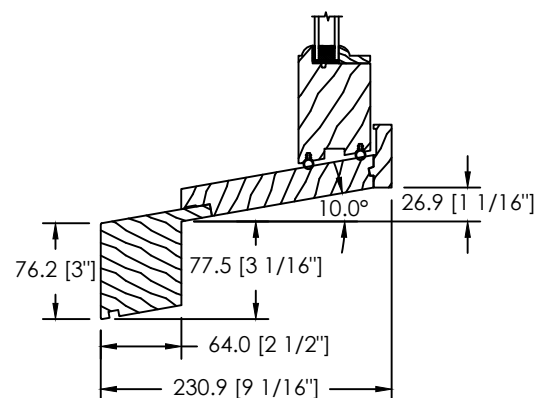
EXTENSION DE SEUIL SPÉCIALE (DS-073)
