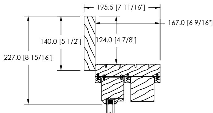
MOULURE À BRIQUE PLATE 140MM (D-118)
