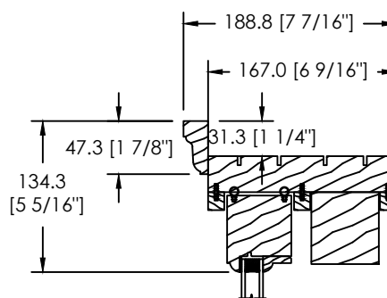
MOULURE À BRIQUE SPÉCIALE (DS-061)
