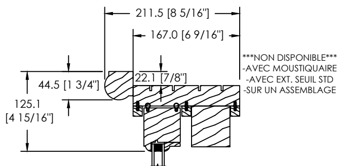
MOULURE À BRIQUE SPÉCIALE (DS-030)
