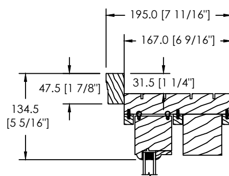
MOULURE À BRIQUE 908 (D-064)
