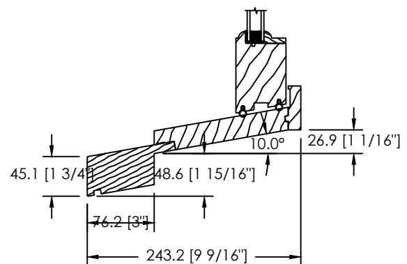
EXTENSION DE SEUIL HISTORIQUE (GB-058)
