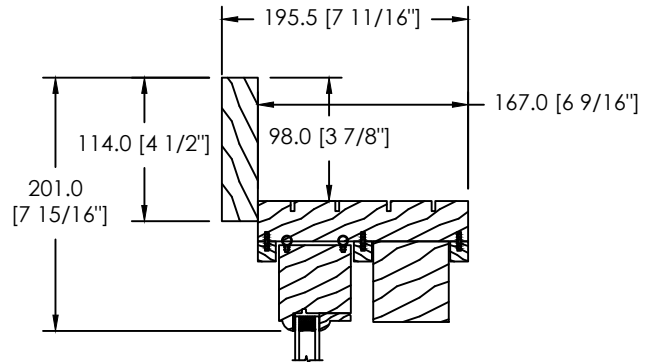
MOULURE À BRIQUE PLATE 114MM (D-117)
