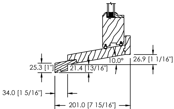
EXTENSION DE SEUIL STANDARD (GB-021)
