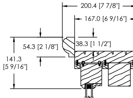
MOULURE À BRIQUE SPÉCIALE (DS-017)
