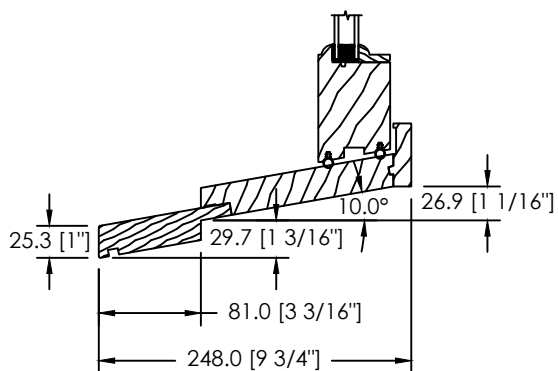
EXTENSION DE SEUIL 76MM (GB-040)
