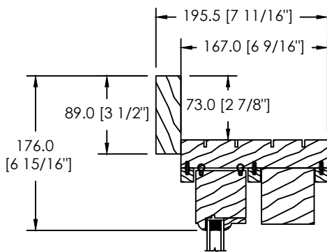
MOULURE À BRIQUE PLATE 89MM (D-061)
