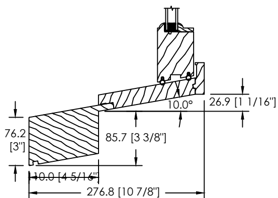
EXTENSION DE SEUIL SPÉCIALE (DS-072)
