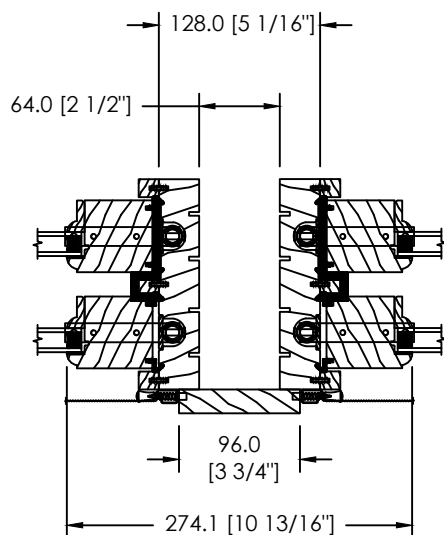
ESPACE MODULAIRE OU STUD POCKET 64MM
