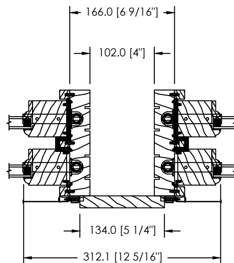
ESPACE MODULAIRE OU STUD POCKET 102MM
