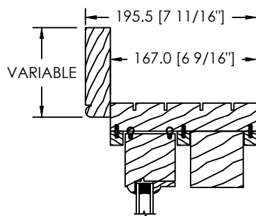
MOULURE À BRIQUE VARIABLE (DS-001)
