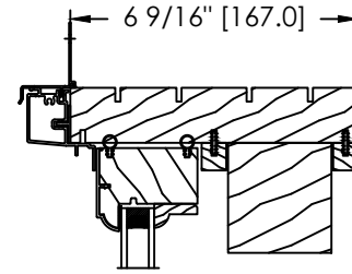
NAILING FIN
