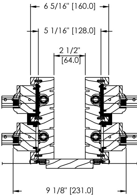
2 1/2" SPACE MULL OR STUD POCKET
