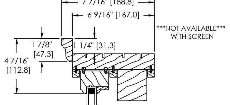
SPECIAL BRICKMOULD (DS-061)
