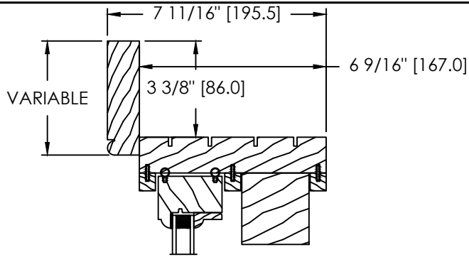
VARIABLE BRICKMOULD (DS-001)
