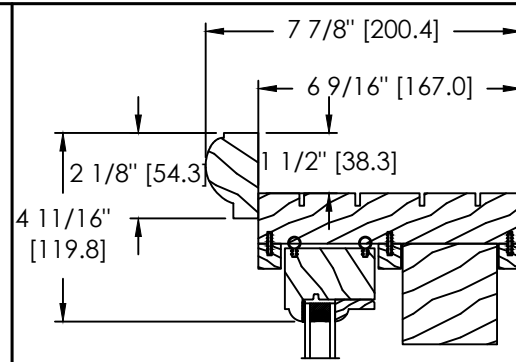
SPECIAL BRICKMOULD (DS-017)
