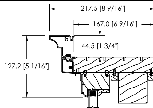
MOULURE À BRIQUE SKYLER
