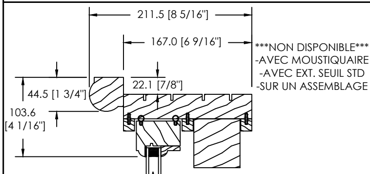
MOULURE À BRIQUE SPÉCIALE (DS-030)
