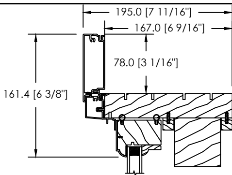
MOULURE À BRIQUE PLATE 89MM
