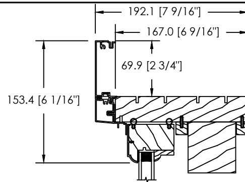
MOULURE À BRIQUE PLATE 70MM
