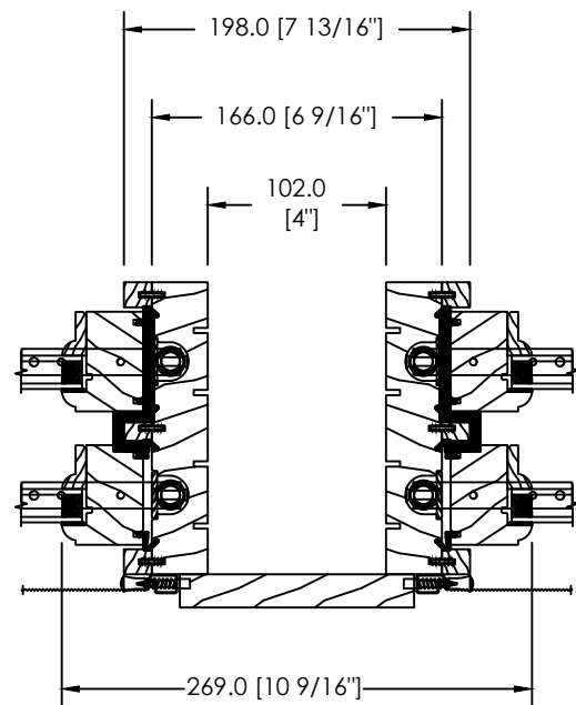
ESPACE MODULAIRE OU STUD POCKET 102MM
