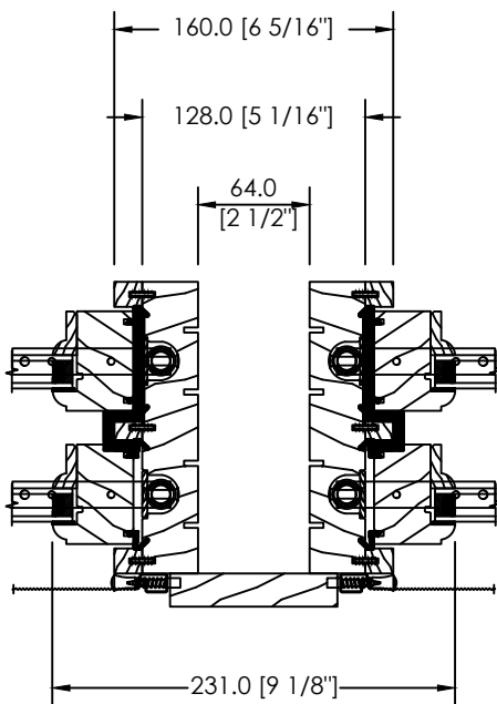
ESPACE MODULAIRE OU STUD POCKET 64MM
