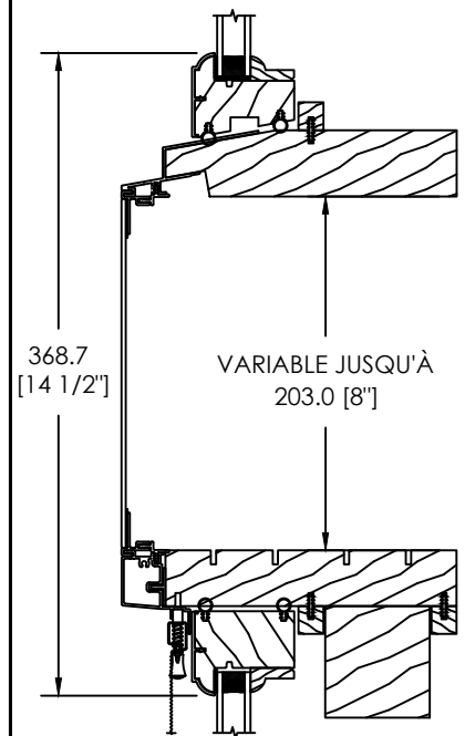
ESPACE MODULAIRE OU STUD POCKET NON STANDARD JUSQU'À 203MM MAXIMUM
