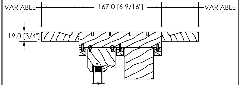
EXTENSION EXT. ET INT. VARIABLE
