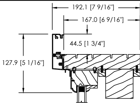
MOULURE À BRIQUE PLATE 44.5MM
