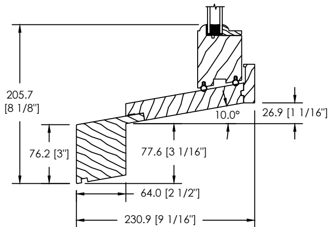
EXTENSION DE SEUIL SPÉCIALE (DS-073)
