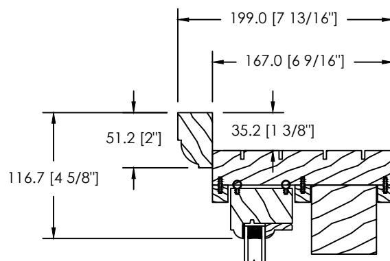
MOULURE À BRIQUE SPÉCIALE (DS-065)
