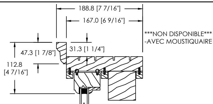
MOULURE À BRIQUE SPÉCIALE (DS-061)
