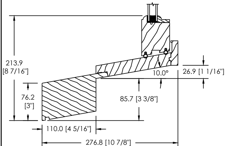
EXTENSION DE SEUIL SPÉCIALE (DS-072)
