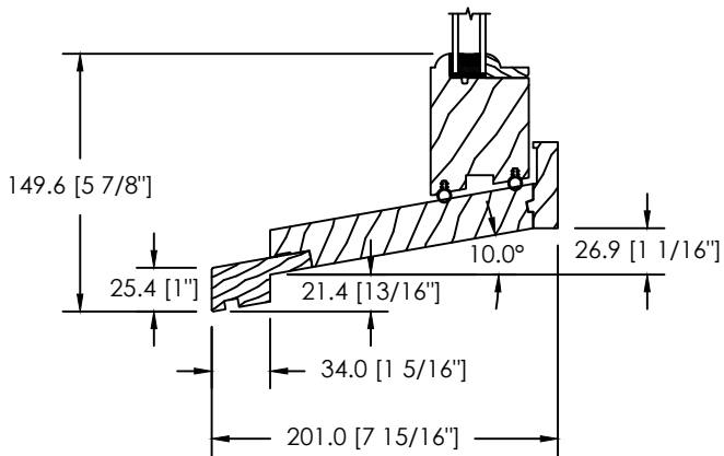
EXTENSION DE SEUIL STANDARD (GB-021)
