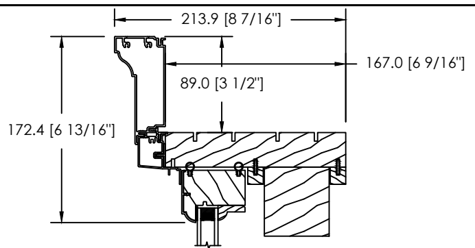
MOULURE À BRIQUE BACK BEND
