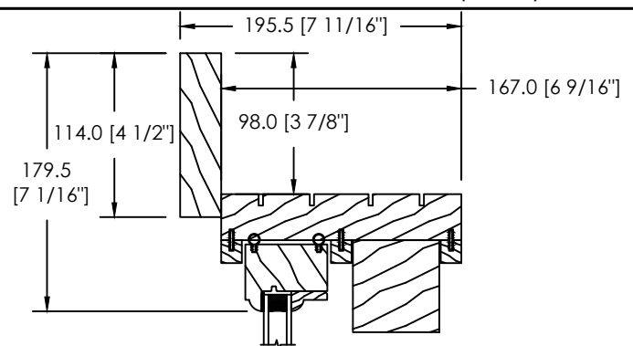
MOULURE À BRIQUE PLATE 114MM (D-117)
