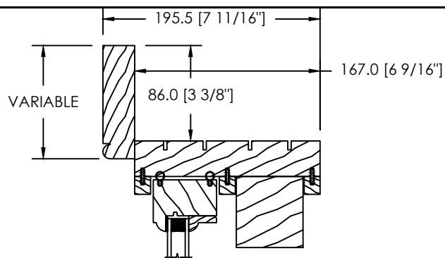
MOULURE À BRIQUE VARIABLE (DS-001)
