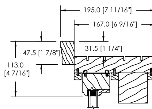
MOULURE À BRIQUE 908 (D-064)
