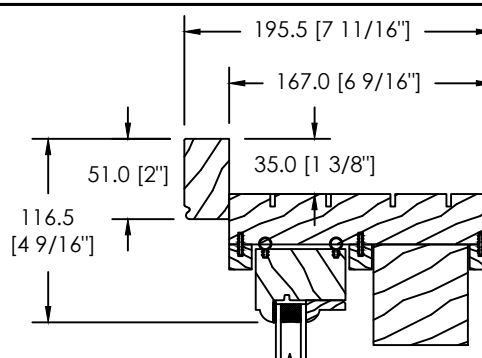
MOULURE À BRIQUE SPÉCIALE (DS-031)
