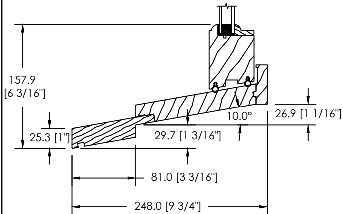
EXTENSION DE SEUIL 76MM (GB-040)
