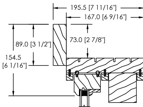
MOULURE À BRIQUE PLATE 89MM (D-061)
