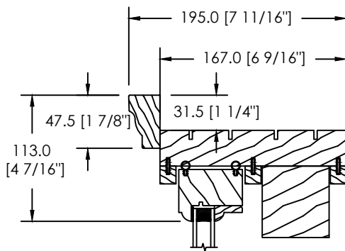
MOULURE À BRIQUE COLONIALE (D-017)
