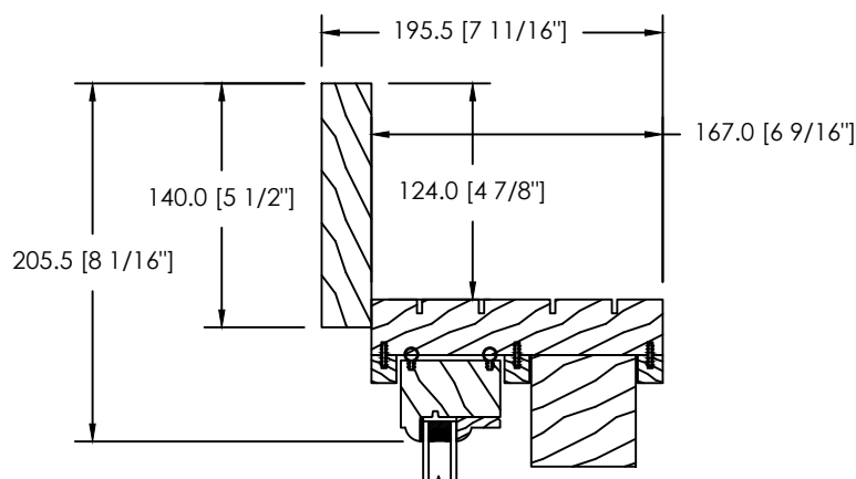
MOULURE À BRIQUE PLATE 140MM (D-118)
