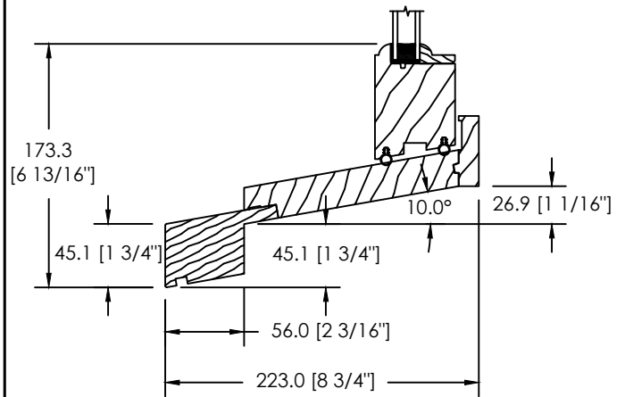
EXTENSION DE SEUIL HISTORIQUE (GB-036)
