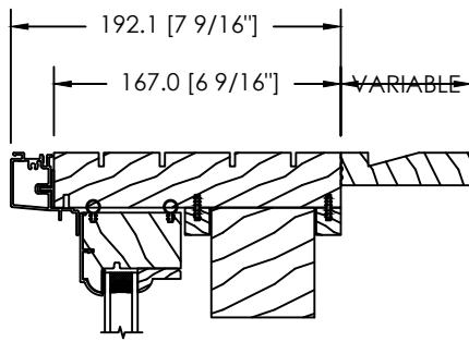
EXTENSION INTÉRIEUR VARIABLE
