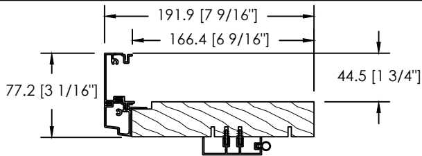
MOULURE À BRIQUE 908
