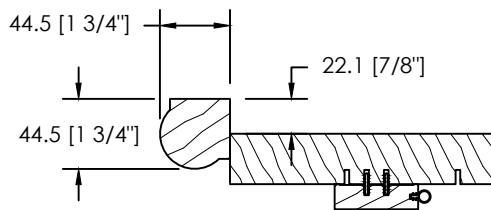
MOULURE À BRIQUE DS-001
