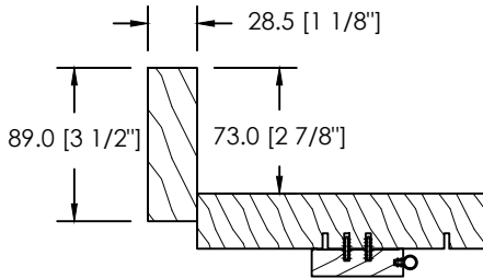
MOULURE À BRIQUE COLONIALE
