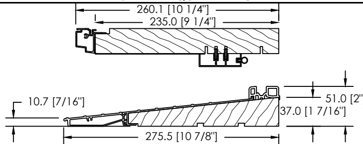
CADRE 235mm - SEUIL ANODISÉ + EXT. 3\"/>
