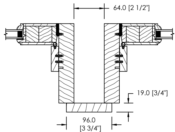
ESPACE MODULAIRE OU STRUCTURAL STANDARD 64mm
