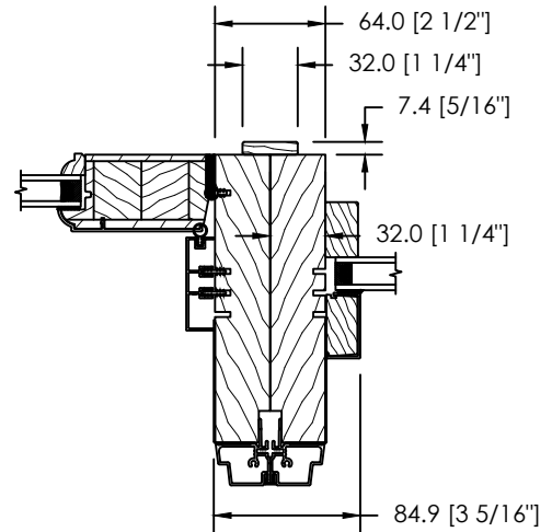
ASSEMBLAGE VERTICAL MODULAIRE AVEC THERMOS FIXE (SL-1)
