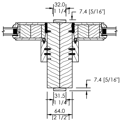
ASSEMBLAGE VERTICAL MODULAIRE
