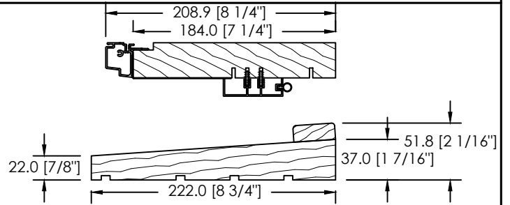
CADRE 184mm - SEUIL EN ACAJOU BRIS THERMIQUE EN ACAJOU
