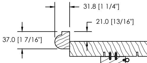
MOULURE À BRIQUE DS-030
