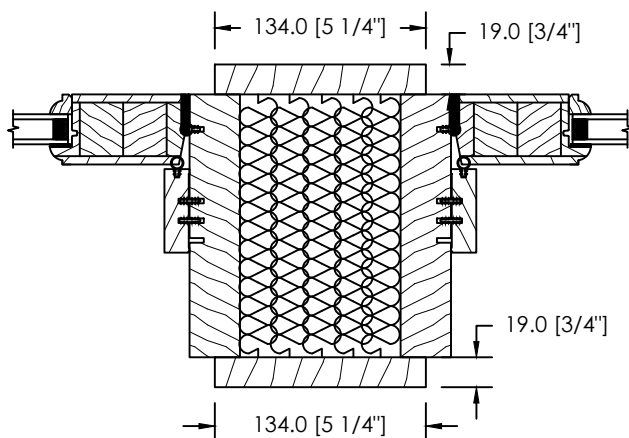
ESPACE MODULAIRE OU STRUCTURAL ISOLÉ - STANDARD 102mm
