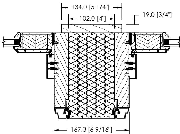
ESPACE MODULAIRE OU STRUCTURAL ISOLÉ - STANDARD 102mm
