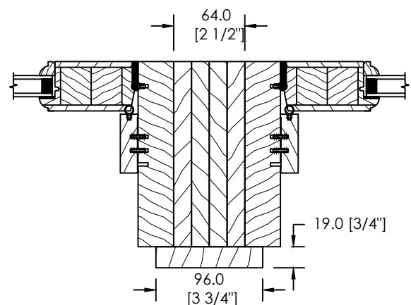
ESPACE MODULAIRE OU STRUCTURAL SOLIDE - STANDARD 64mm
