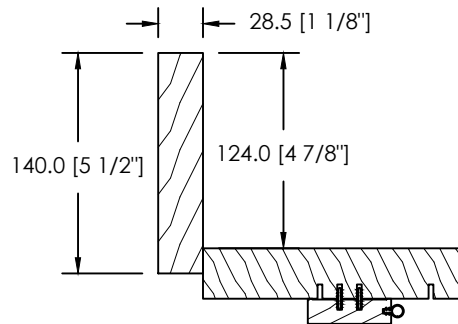
MOULURE À BRIQUE PLATE 140MM
