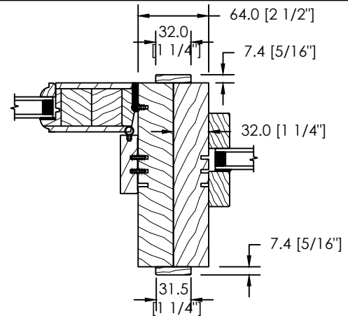
ASSEMBLAGE VERTICAL MODULAIRE AVEC THERMOS FIXE (SL-1)
