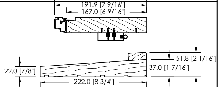
CADRE 167mm - SEUIL EN ACAJOU BRIS THERMIQUE EN ACAJOU
