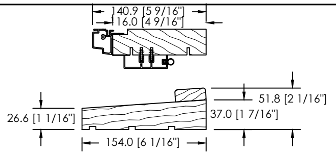
CADRE 116mm - SEUIL EN ACAJOU BRIS THERMIQUE EN ACAJOU
