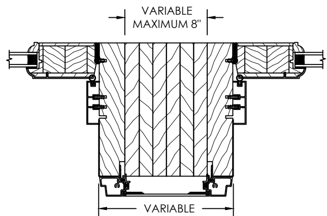
ESPACE MODULAIRE OU STRUCTURAL SOLIDE - NON-STANDARD
