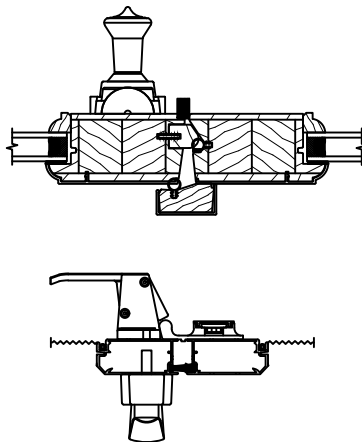
MOUSTIQUAIRE SUR PENTURE AS-09
