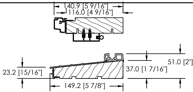
CADRE 116mm - SEUIL ANODISÉ BRIS THERMIQUE EN PVC
