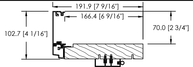
AILE DE CLOUAGE
