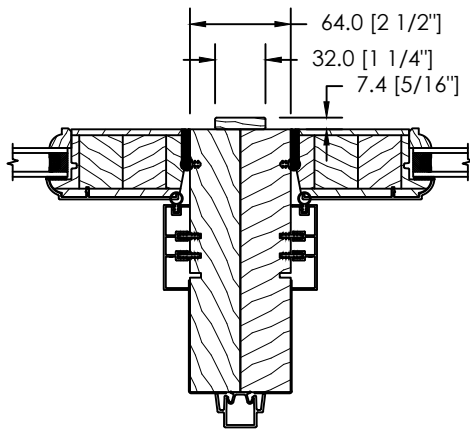
ASSEMBLAGE VERTICAL MODULAIRE
