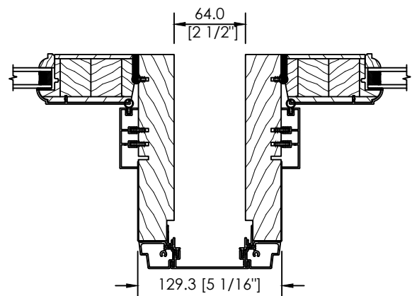
ESPACE MODULAIRE OU STRUCTURAL STANDARD 64mm
