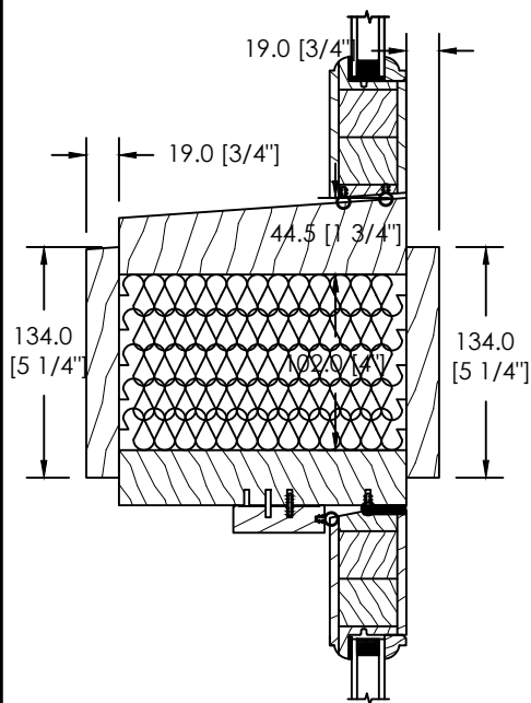
IMPOSTE THERMOS FIXE (TR-1) ASSEMBLAGE MODULAIRE
