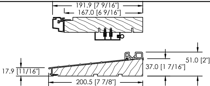
CADRE 167mm - SEUIL ANODISÉ BRIS THERMIQUE EN PVC
