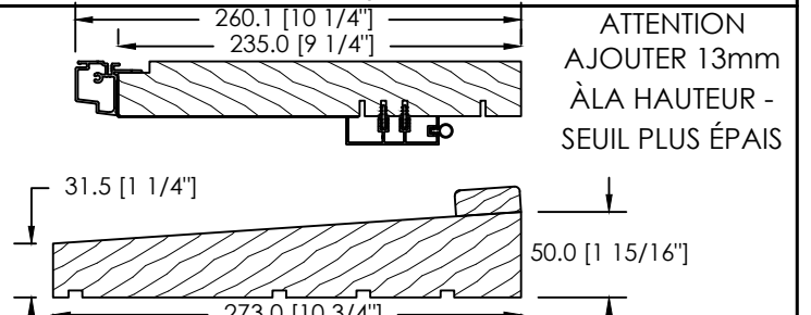
CADRE 235mm - SEUIL EN ACAJOU BRIS THERMIQUE EN ACAJOU
