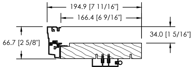
EXTENSION INTÉRIEURE VARIABLE
