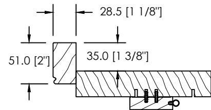
MOULURE À BRIQUE DS-017
