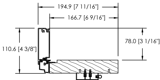
MOULURE À BRIQUE PLATE 44.5MM D-116
