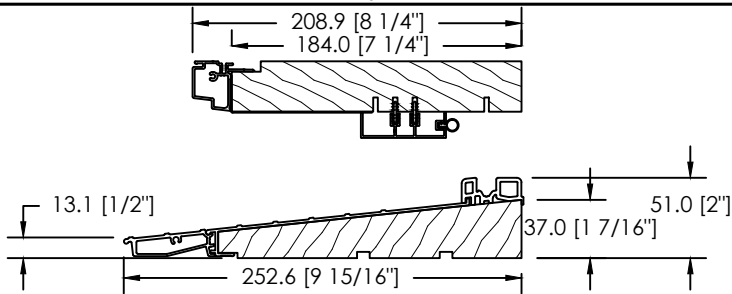
CADRE 184mm - SEUIL ANODISÉ + EXT. 2\"/>
