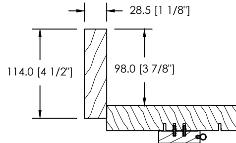
MOULURE À BRIQUE 908
