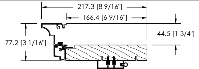
MOULURE À BRIQUE PLATE 70MM D-066
