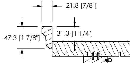
MOULURE À BRIQUE DS-031
