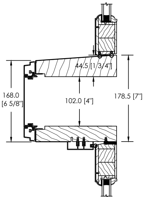
IMPOSTE EN VOLET ASSEMBLAGE MODULAIRE
