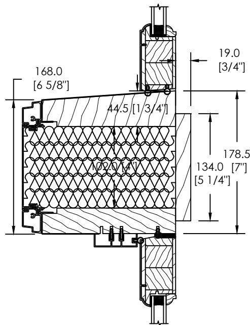
IMPOSTE THERMOS FIXE (TR-1) ASSEMBLAGE MODULAIRE
