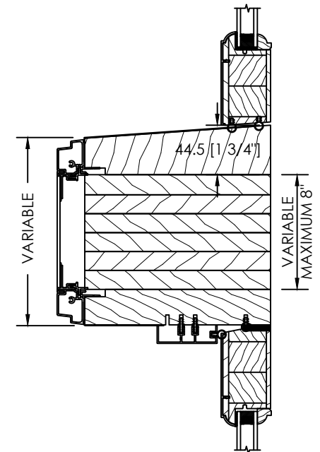
ESPACE MODULAIRE OU STRUCTURAL STANDARD 64mm
