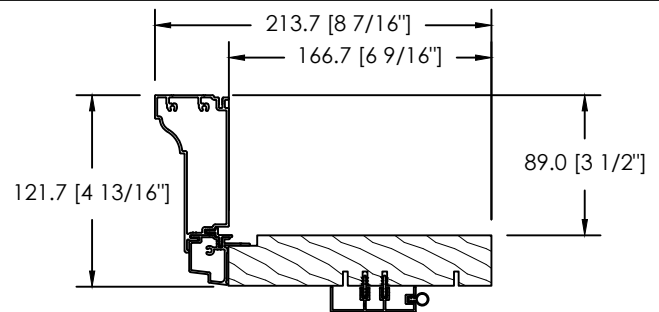
MOULURE À BRIQUE SKYLER D-174
