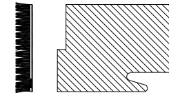
CF-134 Coupe-Froid à Balai pour volet 5" Droit / Brush Weather Strip for Right 5" Sash
