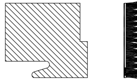
CF-133 Coupe-Froid à Balai pour volet 3 5 / 8 " Gauche / Brush Weather Strip for Left 3 5 / 8 " Sash
