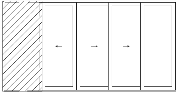
CF-133 Coupe-Froid à Balai pour volet 3 5 / 8 " Gauche / Brush Weather Strip for Left 3 5 / 8 " Sash
