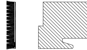
CF-133 Coupe-Froid à Balai pour volet 3 5 / 8 " Droit / Brush Weather Strip for Right 3 5 / 8 " Sash
