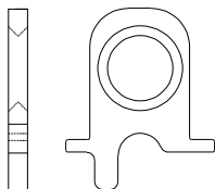
Q-405-A Plaque Structurale de volet avec astragale / Sash Structural Plate with astragal
