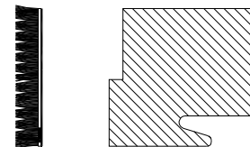
CF-133 Coupe-Froid è Balai pour volet 3 \frac{5}{8} " Droit / Brush Weather Strip for Right 3 \frac{5}{8} " Sash
