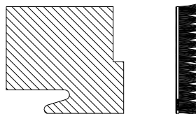
CF-133 Coupe-Froid è Balai pour volet 3 \frac{5}{8} " Gauche / Brush Weather Strip for Left 3 \frac{5}{8} " Sash
