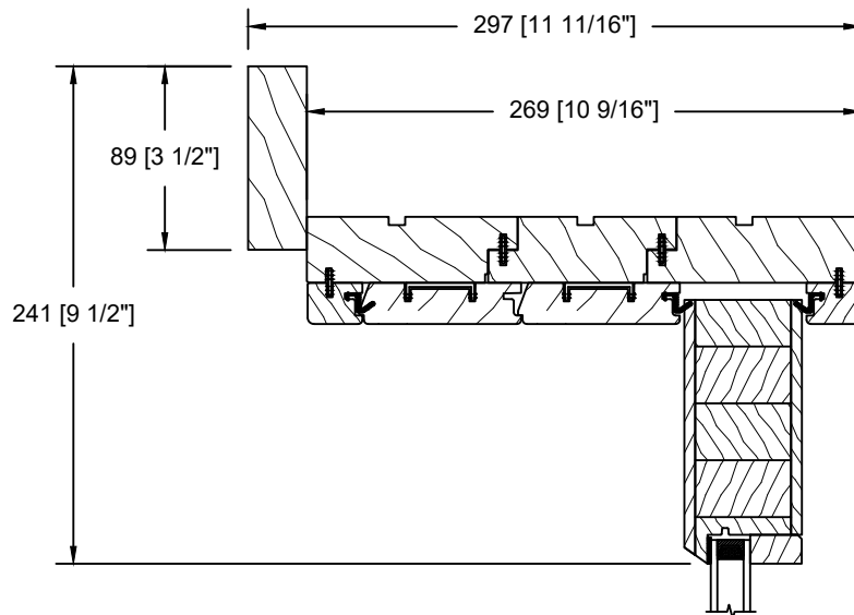
MOULURE À BRIQUE PLATE 3 1/2"
