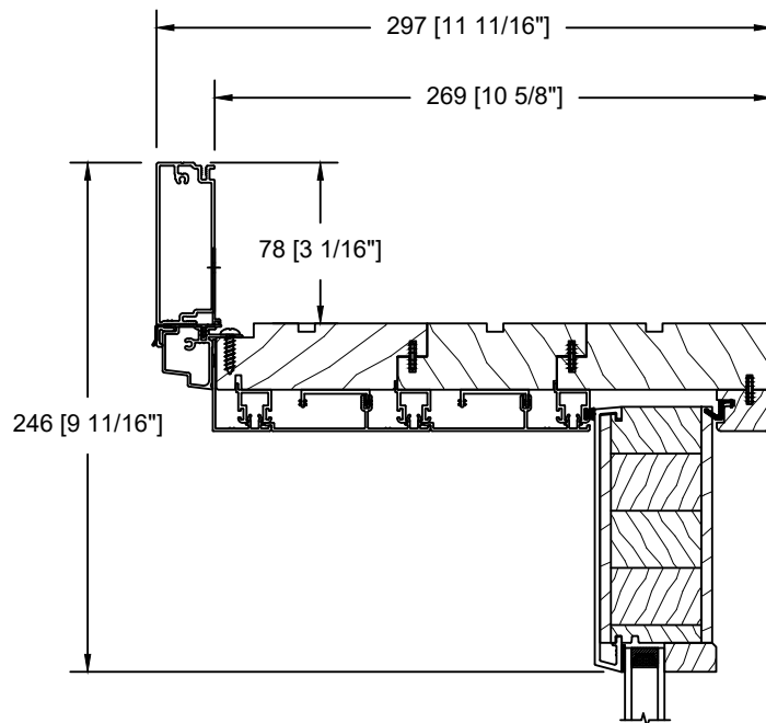
MOULURE À BRIQUE PLATE 3 1/2" (D-050)
