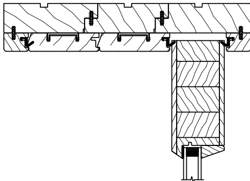
VOLET PUTTY GLAZE ET PARECLOUSE CONTEMPORAINE 5"
