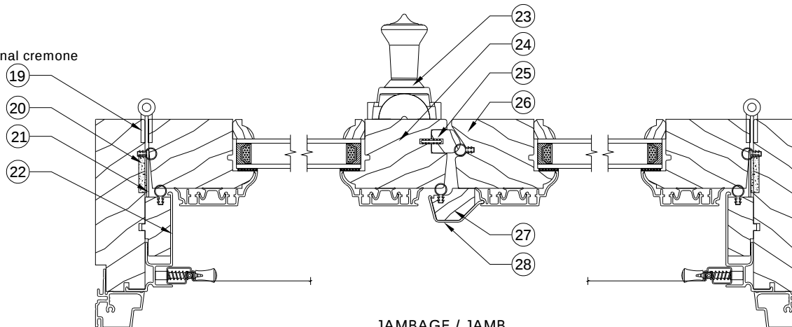
JAMBAGE / JAMB
