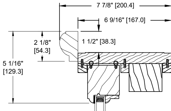
SPECIAL BRICKMOULD (DS-017)
