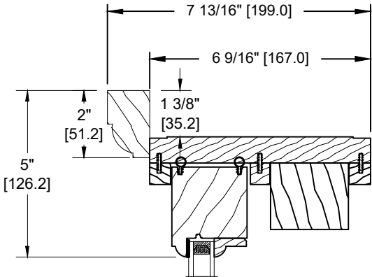
SPECIAL BRICKMOULD (DS-065)
