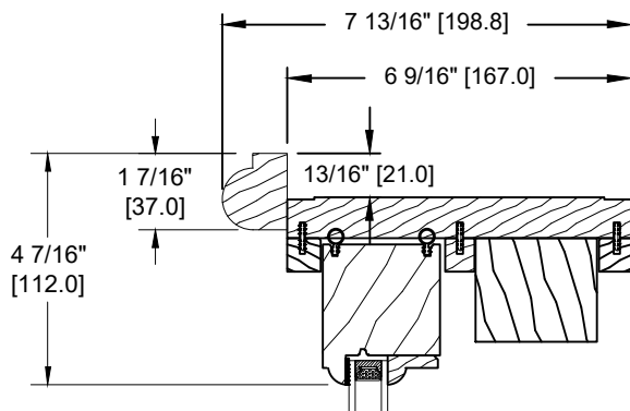
SPECIAL BRICKMOULD (DS-034)
