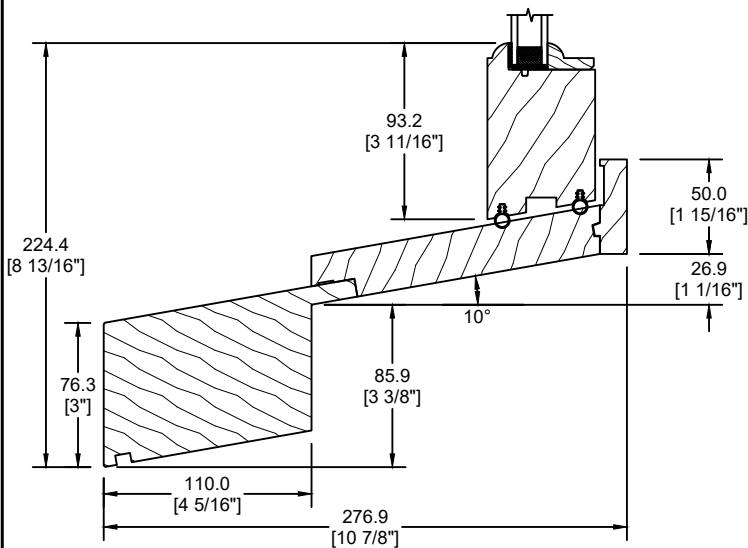
EXTENSION DE SEUIL (DS-072)
