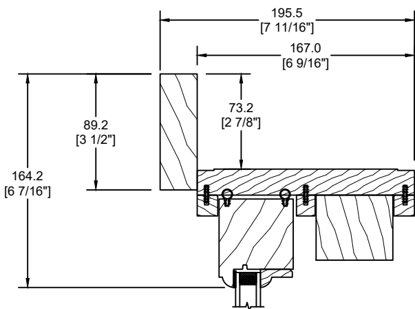
MOULURE À BRIQUE PLATE 89MM (D-061)
