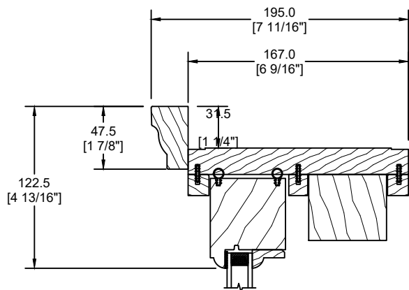
MOULURE À BRIQUE COLONIALE (D-107)
