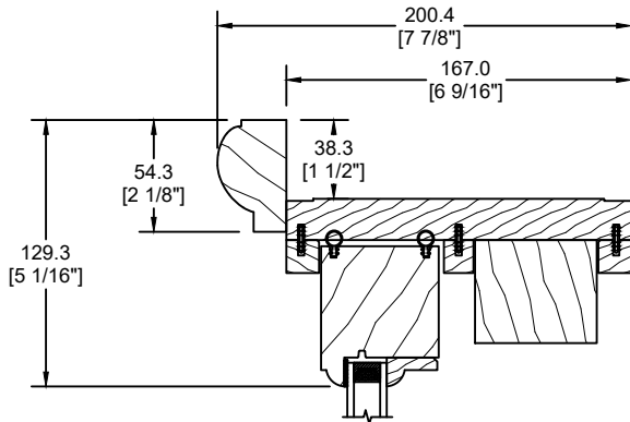
MOULURE À BRIQUE SPÉCIALE (DS-017)
