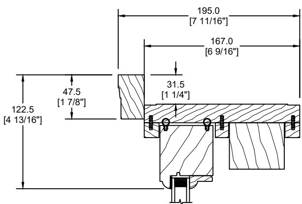
MOULURE À BRIQUE 908 (D-064)
