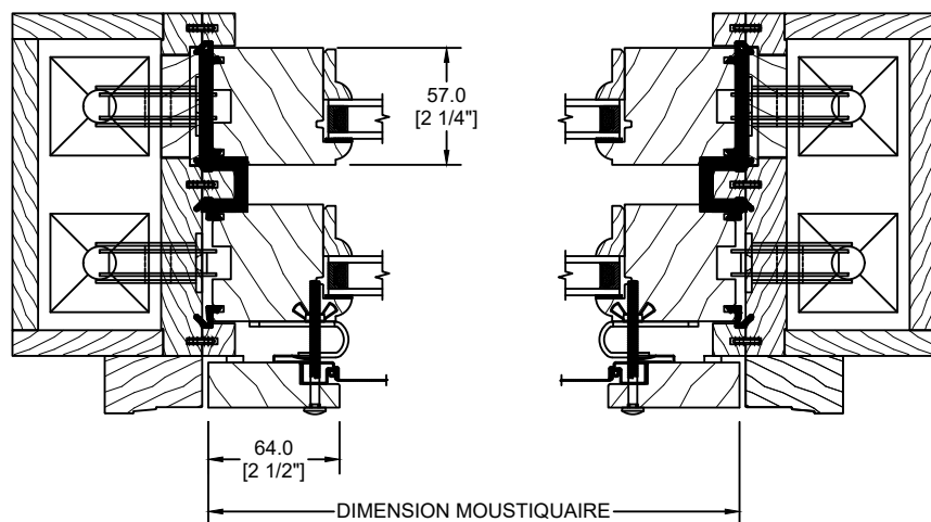
MOUSTIQUAIRE DE BOIS
