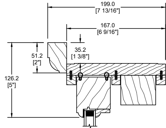
MOULURE À BRIQUE SPÉCIALE (DS-065)
