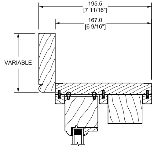
MOULURE À BRIQUE VARIABLE (DS-001)
