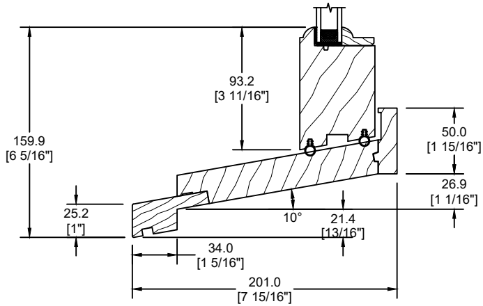
EXTENSION DE SEUIL STANDARD (GB-021)
