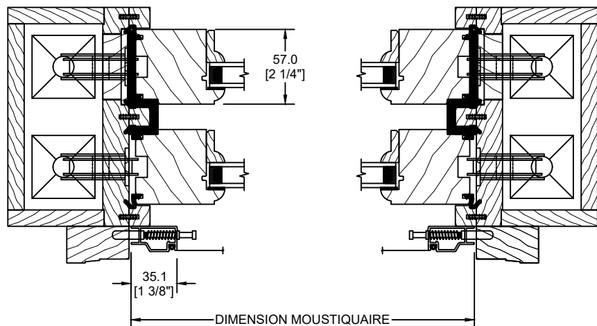
OPTION DEMI-MOUSTIQUAIRE EXTRUDÉE
