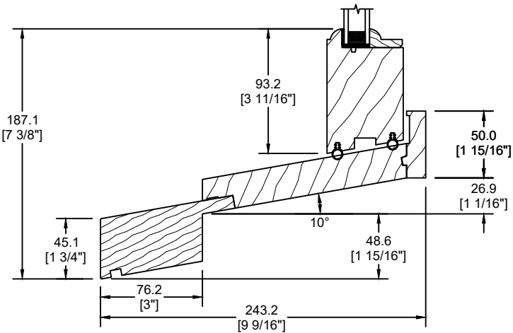
EXTENSION DE SEUIL HISTORIQUE (GB-058)
