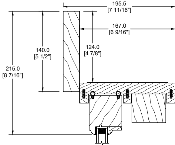
MOULURE À BRIQUE PLATE 140MM (D-118)
