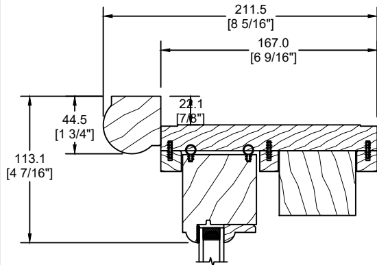
MOULURE À BRIQUE SPÉCIALE (DS-030)
