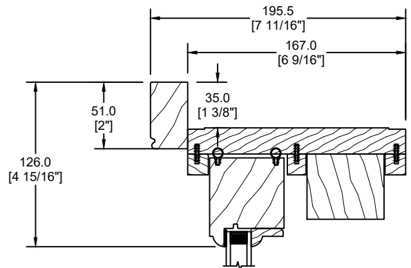
MOULURE À BRIQUE SPÉCIALE (DS-031)
