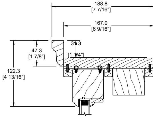
MOULURE À BRIQUE SPÉCIALE (DS-061)
