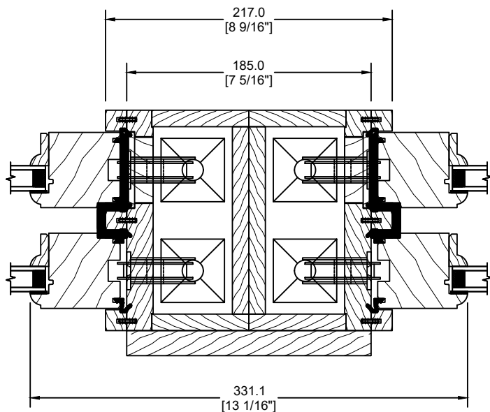
MODULAIRE OPÉRANT
