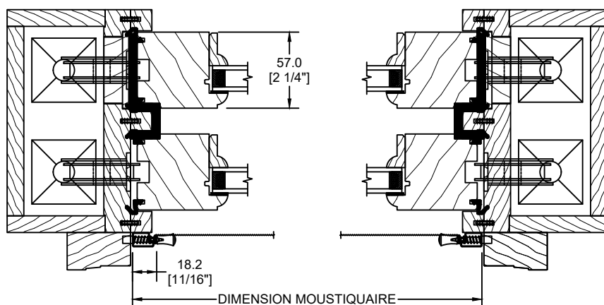
OPTION DEMI-MOUSTIQUAIRE
