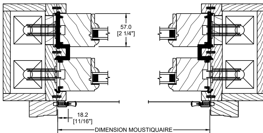
MOUSTIQUAIRE STANDARD
