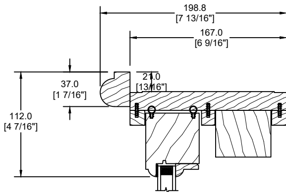
MOULURE À BRIQUE SPÉCIALE (DS-034)
