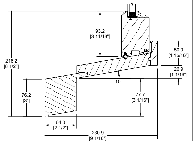
EXTENSION DE SEUIL (DS-073)
