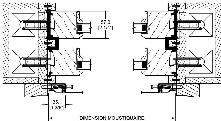
MOUSTIQUAIRE EXTRUDÉE
