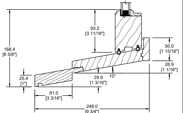
EXTENSION DE SEUIL 76mm (GB-040)
