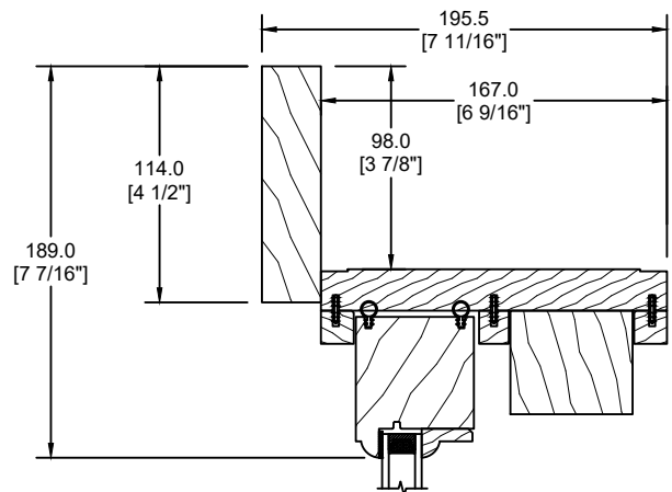
MOULURE À BRIQUE PLATE 114MM (D-117)
