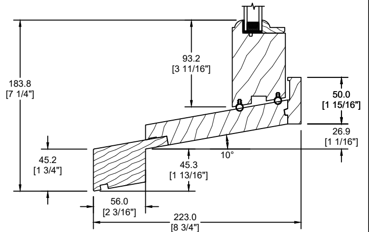
EXTENSION DE SEUIL HISTORIQUE (GB-036)
