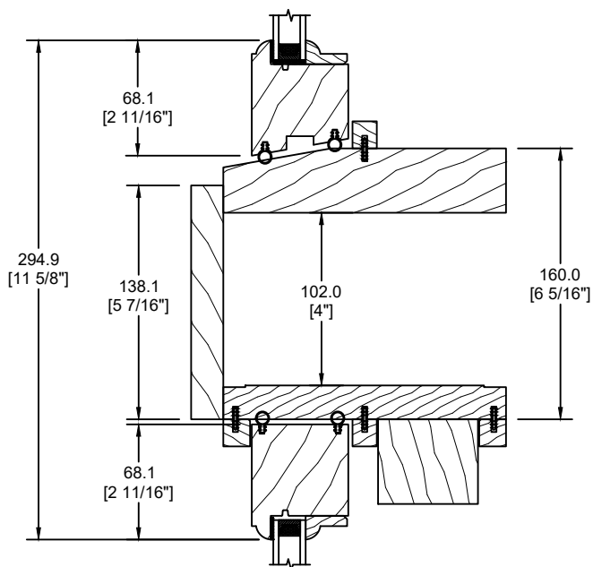
ESPACE MODULAIRE OU STUD POCKET DE 102mm
