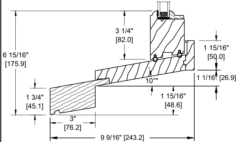
HISTORIC SILL EXTENSION (GB-058)
