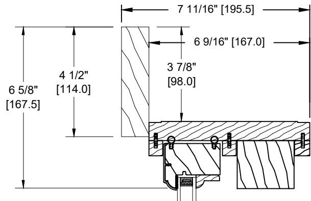
908 BRICKMOULD (D-064)
