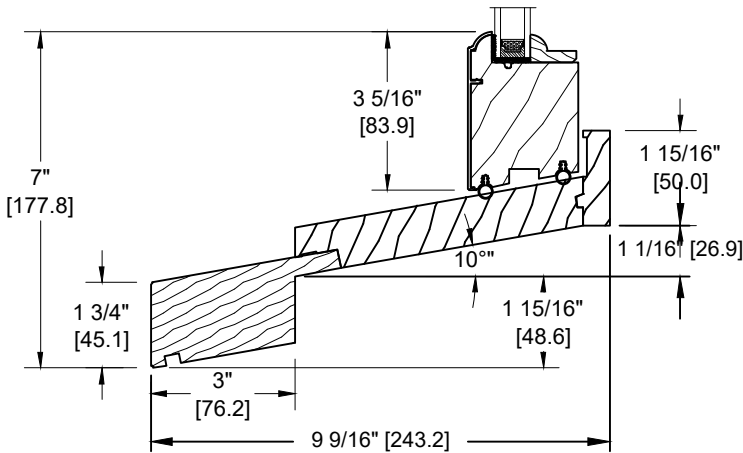
HISTORIC SILL EXTENSION (GB-058)
