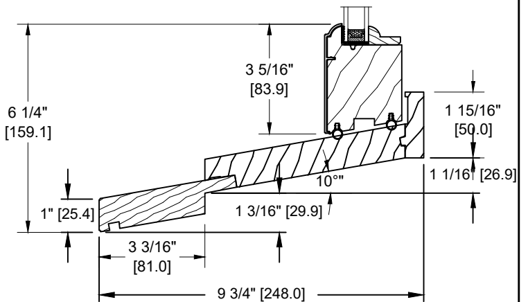
3" SILL EXTENSION (GB-040)
