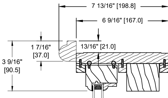
SPECIAL BRICKMOULD (DS-017)
