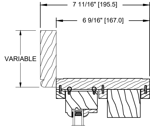
VARIABLE BRICKMOULD (DS-001)
