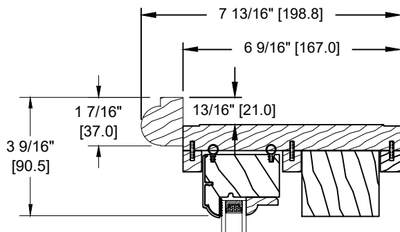
SPECIAL BRICKMOULD (DS-017)
