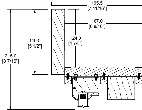
MOULURE À BRIQUE PLATE 140MM (D-118)
