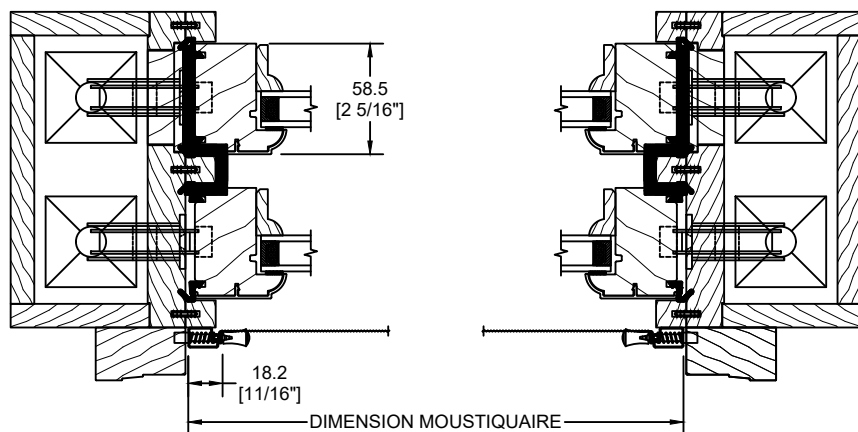
OPTION DEMI-MOUSTIQUAIRE
