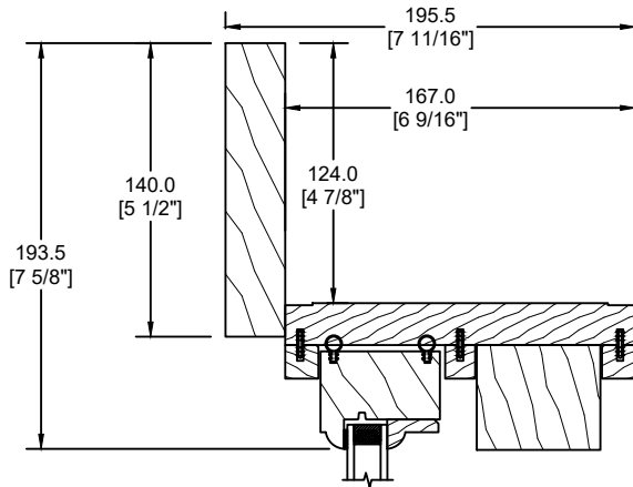
MOULURE À BRIQUE PLATE 140MM (D-118)
