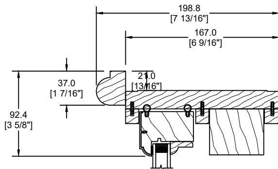
MOULURE À BRIQUE SPÉCIALE (DS-017)
