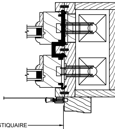
MOUSTIQUAIRE STANDARD
