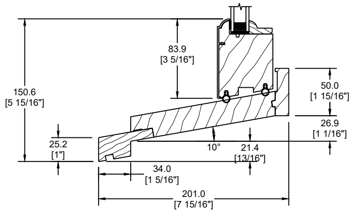
EXTENSION DE SEUIL STANDARD (GB-021)
