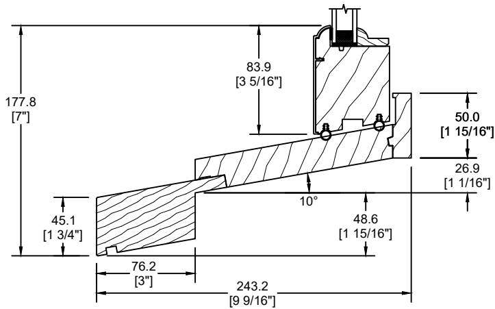
EXTENSION DE SEUIL HISTORIQUE (GB-058)
