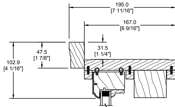
EXTENSION EXT. ET INT. VARIABLE
