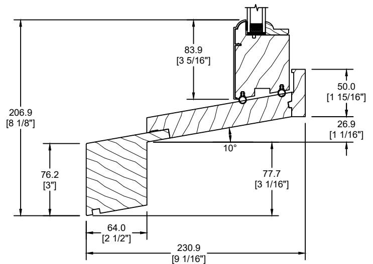
EXTENSION DE SEUIL (DS-073)
