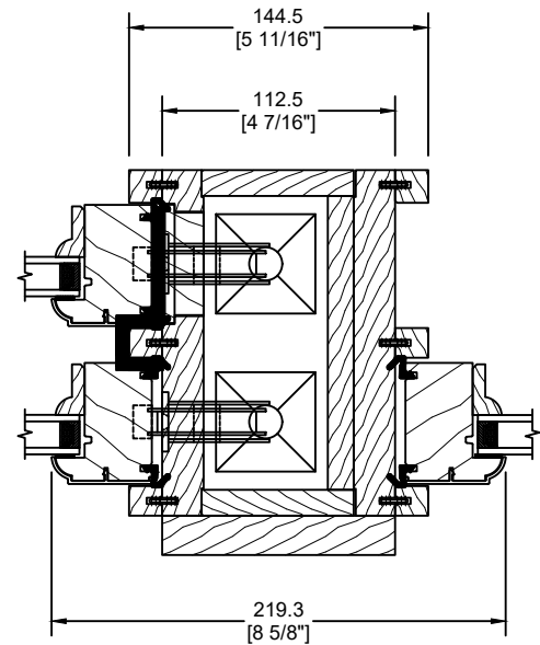
OPÉRANT ET VOLET FIXE
