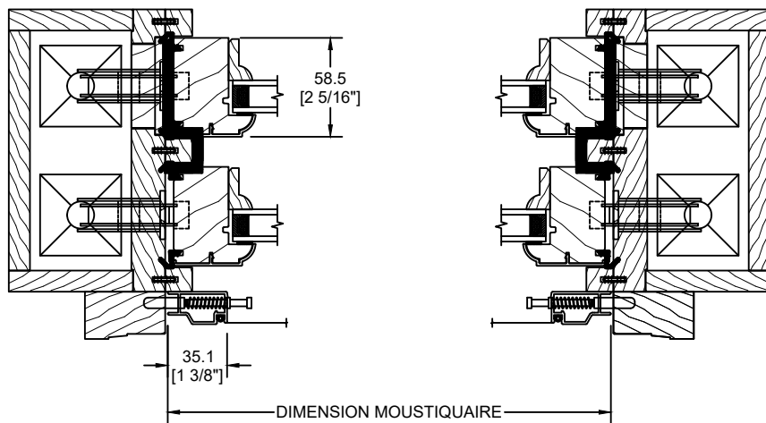
MOUSTIQUAIRE EXTRUDÉE
