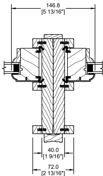
MODULAIRE VOLET FIXE
