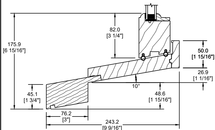
EXTENSION DE SEUIL HISTORIQUE (GB-058)
