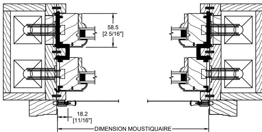
MOUSTIQUAIRE STANDARD
