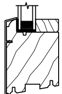
VOLET CONTEMPORAIN & PARECLOSE CARRÉ
