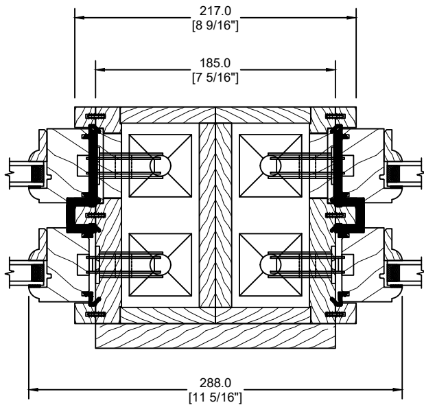
MODULAIRE OPÉRANT
