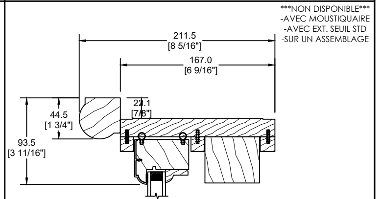
MOULURE À BRIQUE VARIABLE (DS-001)
