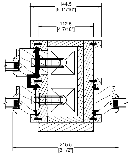
OPÉRANT ET VOLET FIXE
