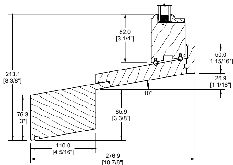
EXTENSION DE SEUIL (DS-072)
