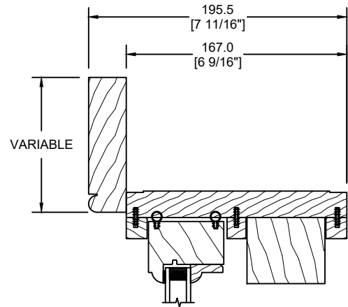
MOULURE À BRIQUE VARIABLE (DS-001)
