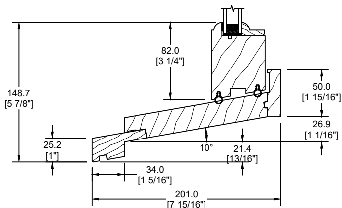
EXTENSION DE SEUIL STANDARD (GB-021)
