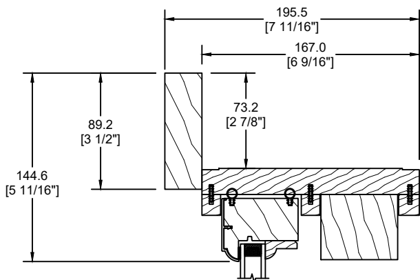
MOULURE À BRIQUE COLONIALE (D-107)
