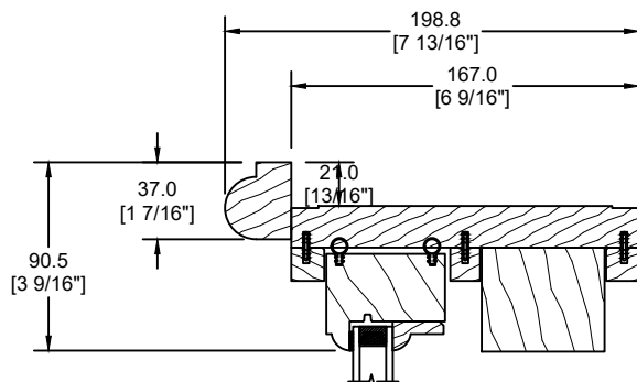
MOULURE À BRIQUE SPÉCIALE (DS-017)
