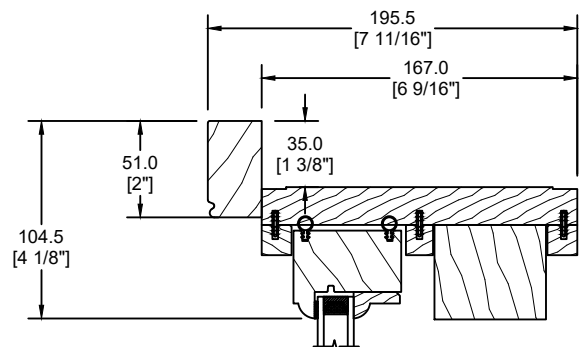
MOULURE À BRIQUE SPÉCIALE (DS-030)
