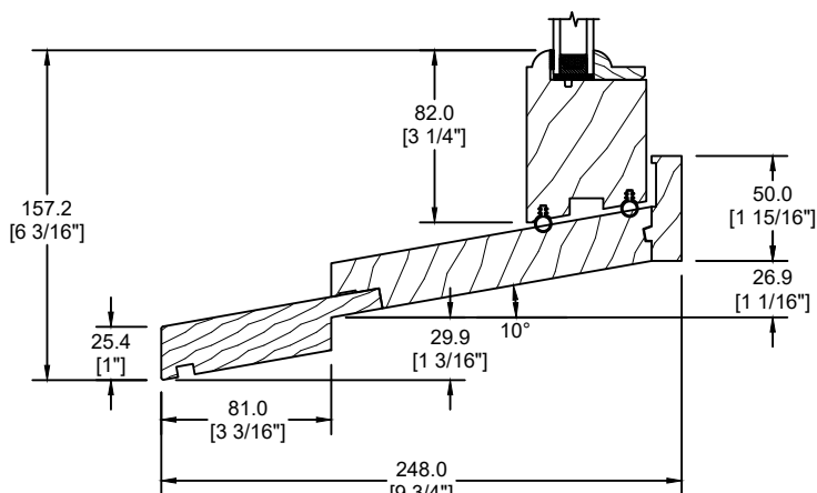
EXTENSION DE SEUIL 76mm (GB-040)
