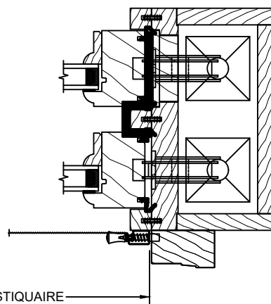
OPTION DEMI-MOUSTIQUAIRE
