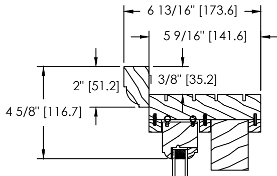
SPECIAL BRICKMOULD (DS-065)
