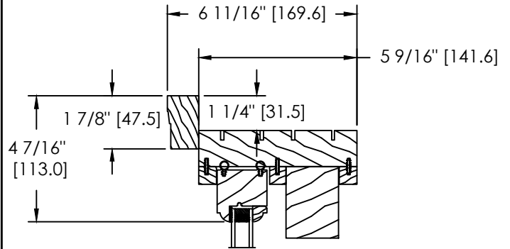
908 BRICKMOULD (D-064)
