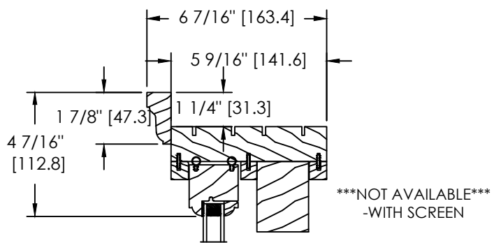
SPECIAL BRICKMOULD (DS-061)
