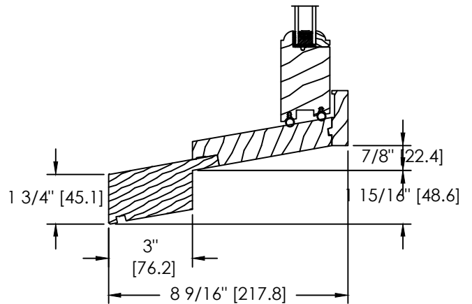
HISTORIC SILL EXTENSION (GB-058)
