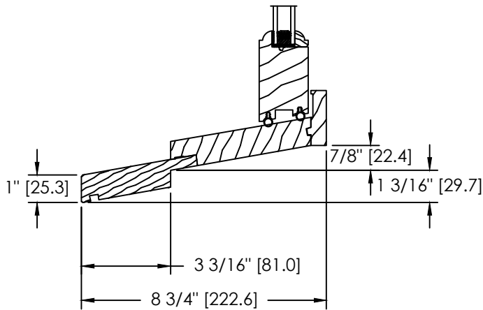
3" SILL EXTENSION (GB-040)
