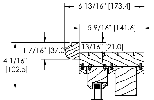
SPECIAL BRICKMOULD (DS-034)
