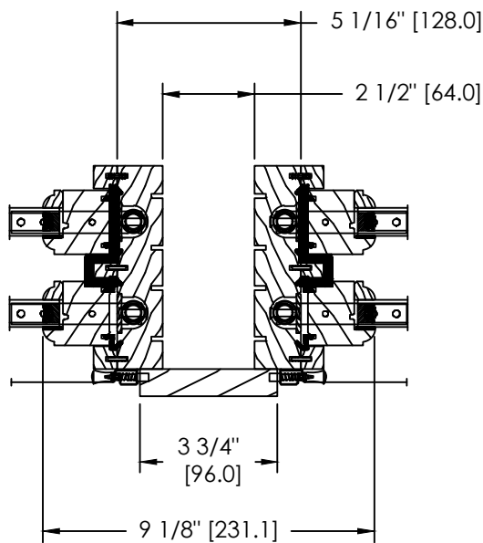
2 1/2" SPACE MULL OR STUD POCKET
