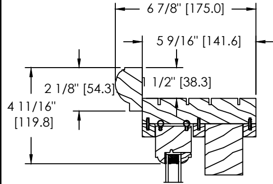
SPECIAL BRICKMOULD (DS-017)
