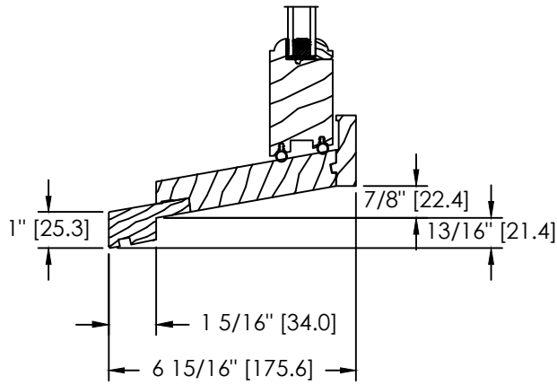
STANDARD SILL EXTENSION (GB-021)
