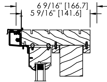
NAILING FIN
