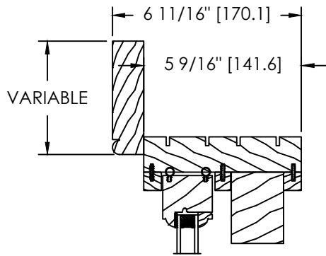
VARIABLE BRICKMOULD (DS-001)
