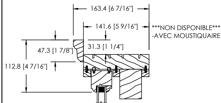
MOULURE À BRIQUE SPÉCIALE (DS-061)
