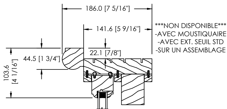
MOULURE À BRIQUE SPÉCIALE (DS-030)
