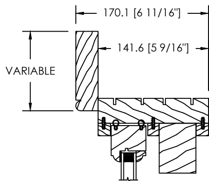
MOULURE À BRIQUE VARIABLE (DS-001)
