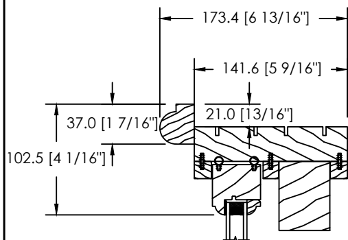
MOULURE À BRIQUE SPÉCIALE (DS-034)
