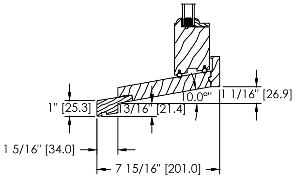
STANDARD SILL EXTENSION (GB-021)
