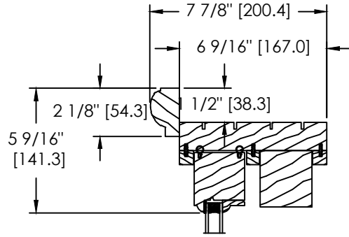
SPECIAL BRICKMOULD (DS-017)
