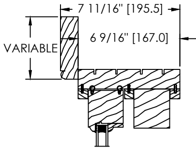
VARIABLE BRICKMOULD (DS-001)
