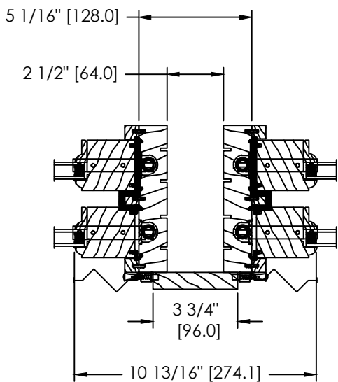
2 1/2" SPACE MULL OR STUD POCKET
