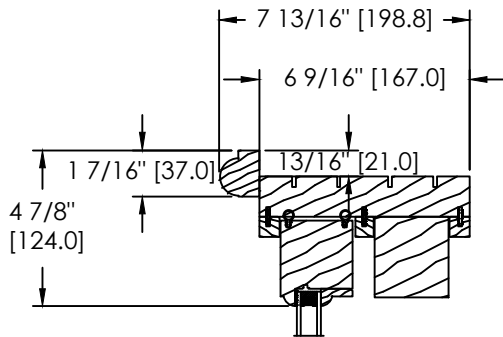
SPECIAL BRICKMOULD (DS-034)
