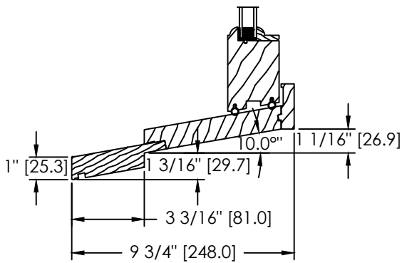
3" SILL EXTENSION (GB-040)
