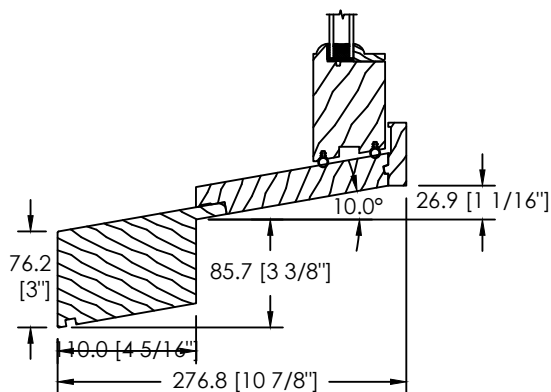
EXTENSION DE SEUIL SPÉCIALE (DS-072)
