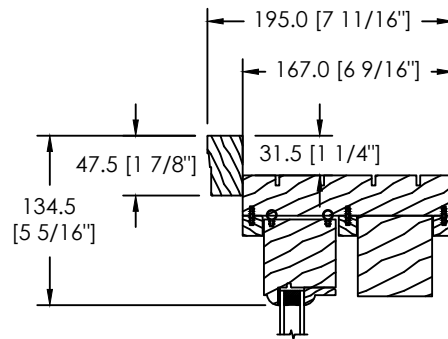
MOULURE À BRIQUE 908 (D-064)
