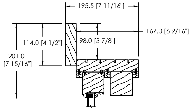
MOULURE À BRIQUE PLATE 114MM (D-117)
