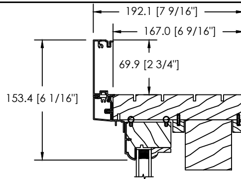
MOULURE À BRIQUE PLATE 70MM
