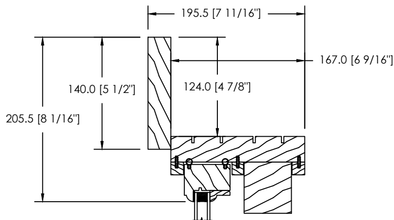
MOULURE À BRIQUE PLATE 140MM (D-118)
