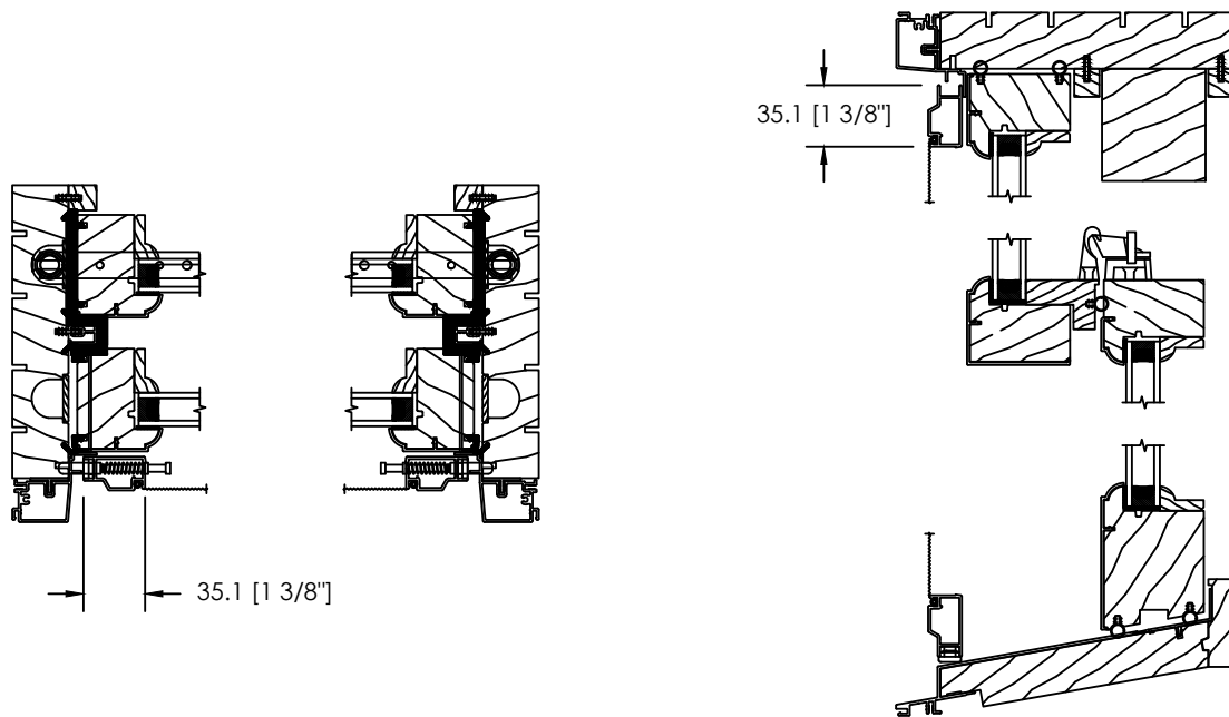
OPTION MOUSTIQUAIRE EXTRUDÉE
