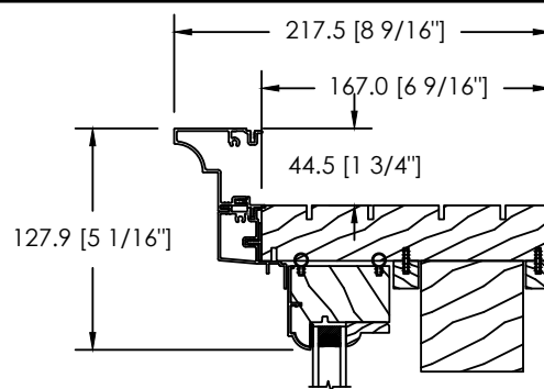
MOULURE À BRIQUE SKYLER
