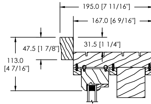
MOULURE À BRIQUE 908 (D-064)
