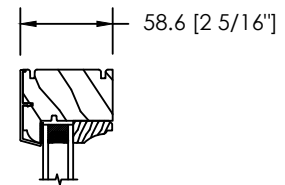
VOLET CONTEMPORAIN & PARECLOUSE CARRÉ
