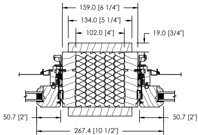
ESPACE MODULAIRE & STRUCTURAL ISOLÉ 102MM
