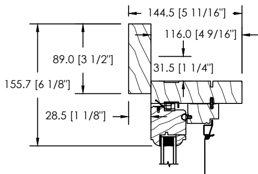
MOULURE À BRIQUE PLATE 89MM
