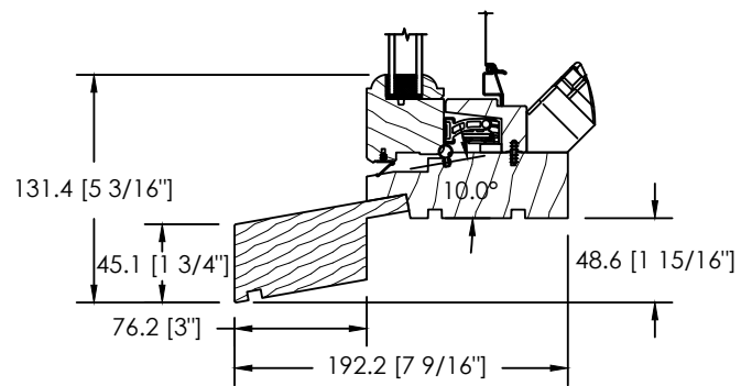
EXTENSION DE SEUIL HISTORIQUE LONG GB-058
