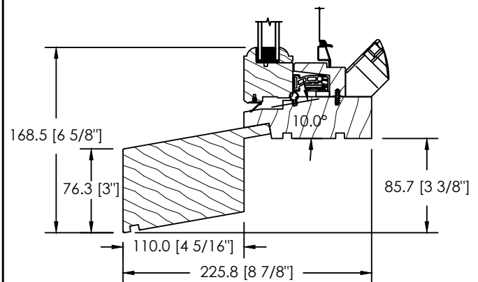
EXTENSION DE SEUIL DS-072
