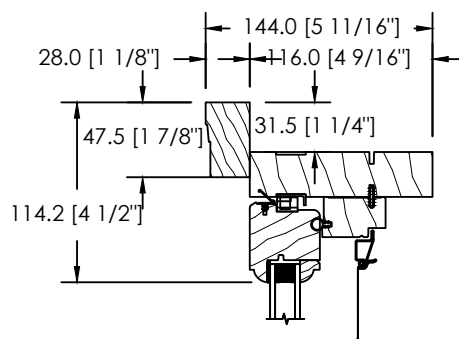
MOULURE À BRIQUE 908
