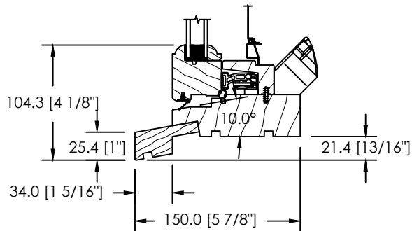
EXTENSION DE SEUIL STANDARD GB-021
