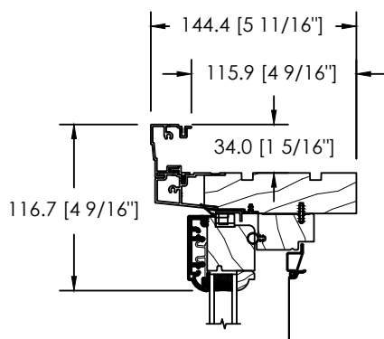
MOULURE À BRIQUE 908
