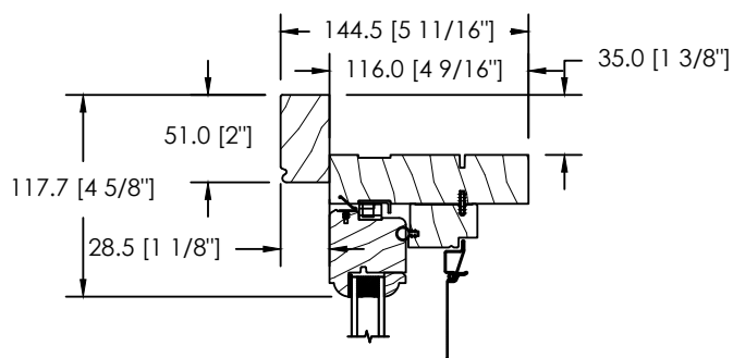
MOULURE À BRIQUE DS-031
