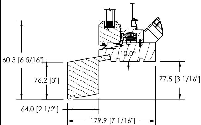
EXTENSION DE SEUIL DS-073
