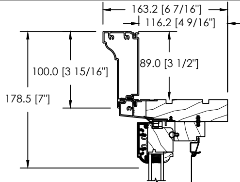
MOULURE À BRIQUE BACK BEND D-090
