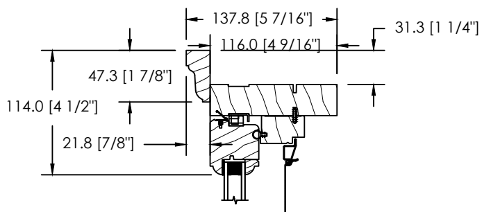
MOULURE À BRIQUE DS-061
