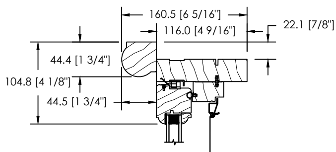
MOULURE À BRIQUE DS-030
