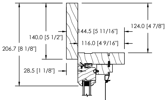
MOULURE À BRIQUE PLATE 140MM
