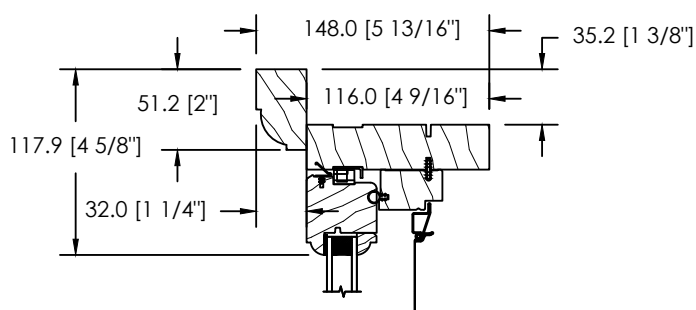
MOULURE À BRIQUE DS-065
