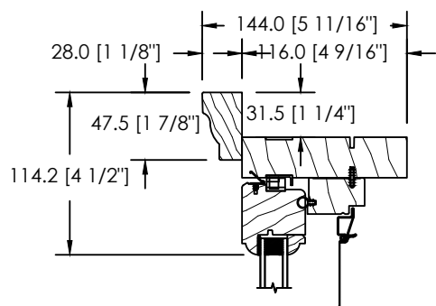
MOULURE À BRIQUE COLONIALE
