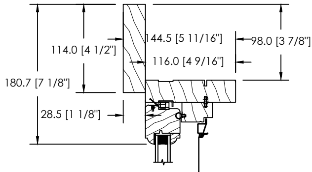
MOULURE À BRIQUE PLATE 114MM
