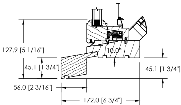
EXTENSION DE SEUIL HISTORIQUE GB-036
