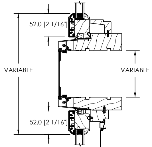
ESPACE MODULAIRE & STRUCTURAL NON-STANDARD 8" MAXIMUM
