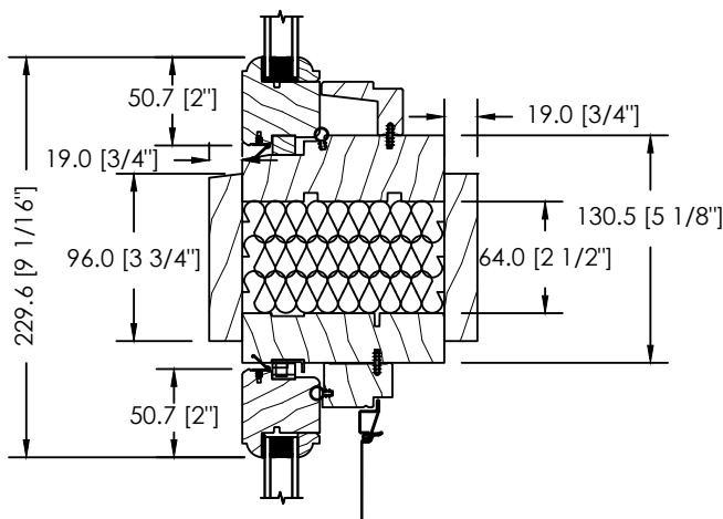
ESPACE MODULAIRE & STRUCTURAL ISOLÉ 64MM
