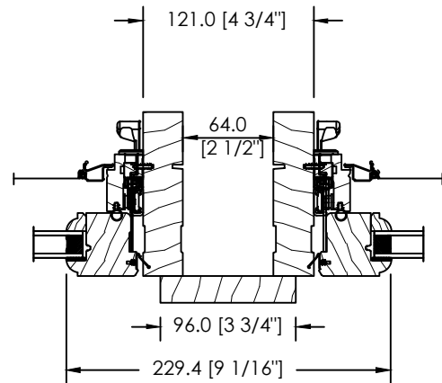
2 1/2" SPACE MULL OR STUD POCKET
