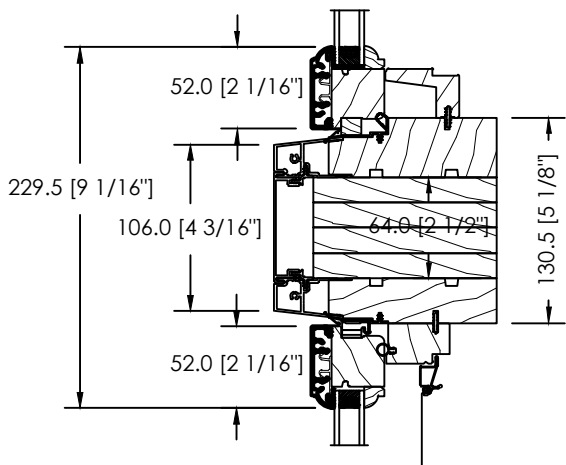
2 1/2" SOLID SPACE MULL OR STUD POCKET
