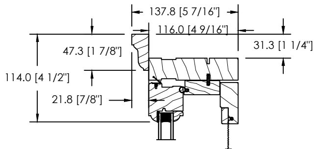
DS-061 BRICKMOULD
