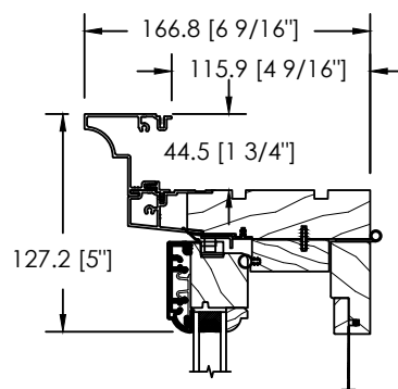
MOULURE À BRIQUE SKYLER D-174
