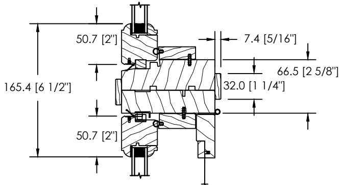
IMPOSTE AVEC VOLET
