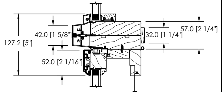
IMPOSTE THERMOS FIXE
