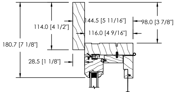
MOULURE À BRIQUE PLATE 114MM
