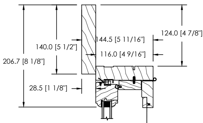
MOULURE À BRIQUE PLATE 140MM
