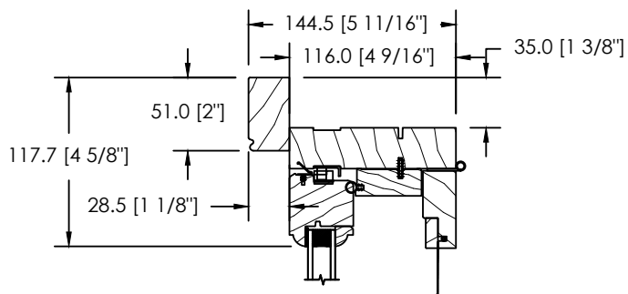
MOULURE À BRIQUE DS-031
