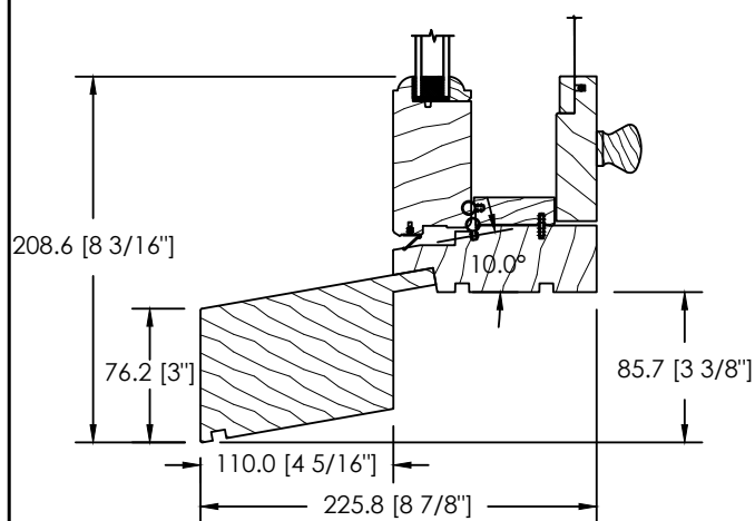
EXTENSION DE SEUIL DS-072
