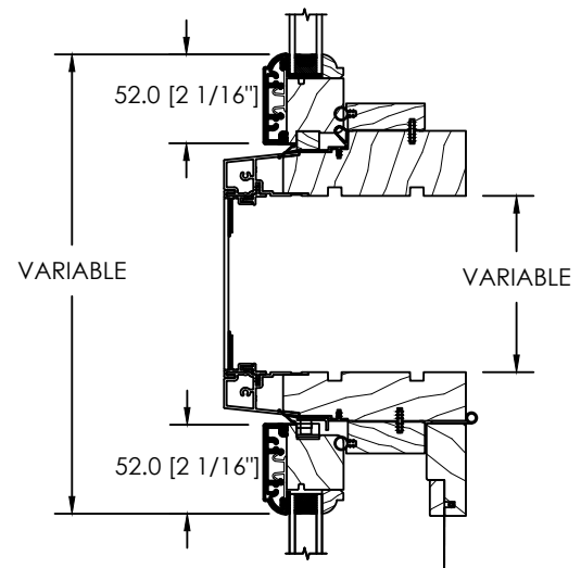
ESPACE MODULAIRE & STRUCTURAL NON-STANDARD 8" MAXIMUM
