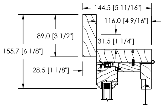
MOULURE À BRIQUE PLATE 89MM
