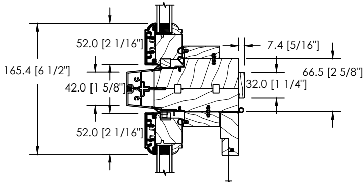
IMPOSTE AVEC VOLET
