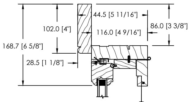
MOULURE À BRIQUE DS-001
