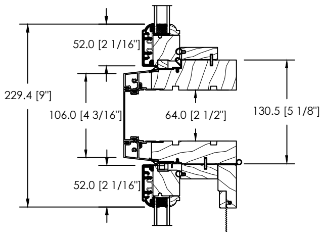
2 1/2" SPACE MULL OR STUD POCKET
