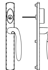
Q-315 Poignée Patio Contemporaine / Contemporary Sliding Handle
