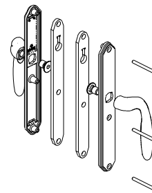
Q-128 Poignée Patio Traditionnelle / Traditionnelle Sliding Handle
