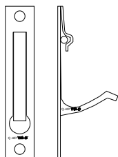
Q-315 Poignée Tirante Encastrée / Edge Door Pull
