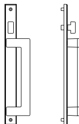
Q-358 Poignée Patio Contemporaine carrée / Square Contemporary Sliding Handle
